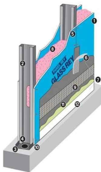
Fig. 3.17. Composición estándar muro de panel de fibrocemento (REY, 2016).
