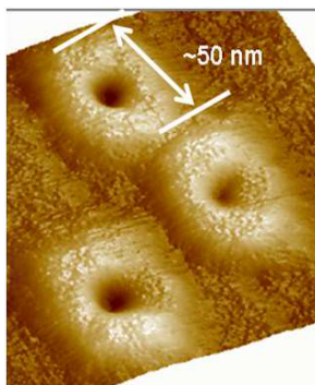
Figura 1.2: Imagen de anillos cuánticos de GaInAs crecidos por MBE, usando el modo de crecimiento Stranski-Krastanov (Axel Lorke et. al. ) [5].
