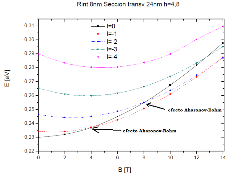
Figura 3.3: Estados confinados con momento angular negativo, para anillos con sección transversal elíptica de R_{ext} - R_{int} = 32 \text{ nm} - 8 \text{ nm} = 24 \text{ nm} y altura 4.8 nm.
