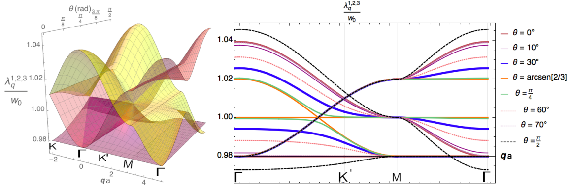
Figura 4.5: Dispersión de plasmones colectiva tridimensional y proyección bidimensional para \varphi = 0 .
