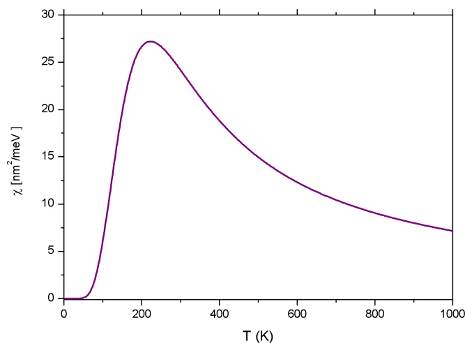
Figura 2.1: Susceptibilidad eléctrica en función de la temperatura, de la distribución de QDs de radio 15nm bajo acción de campos eléctrico E_{mol} = 1\text{meV/nm} y E_{ext} = E_{ef} = 1\text{meV/nm} .
