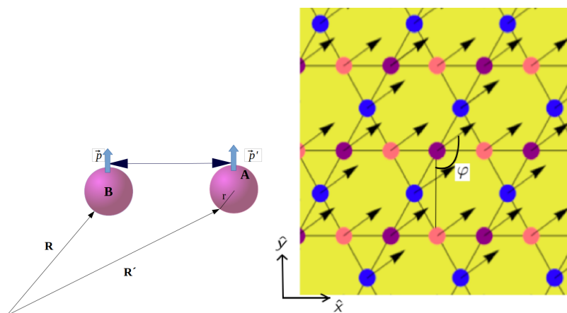
Figura 4.2: Izq. Interacción de dos dipolos puntuales \mathbf{p} y \mathbf{p}' . Der. Red Kagomé infinita de nanopartículas metálicas, con momentos dipolares oscilatorios. (Se muestra el ángulo \varphi en el plano.)
