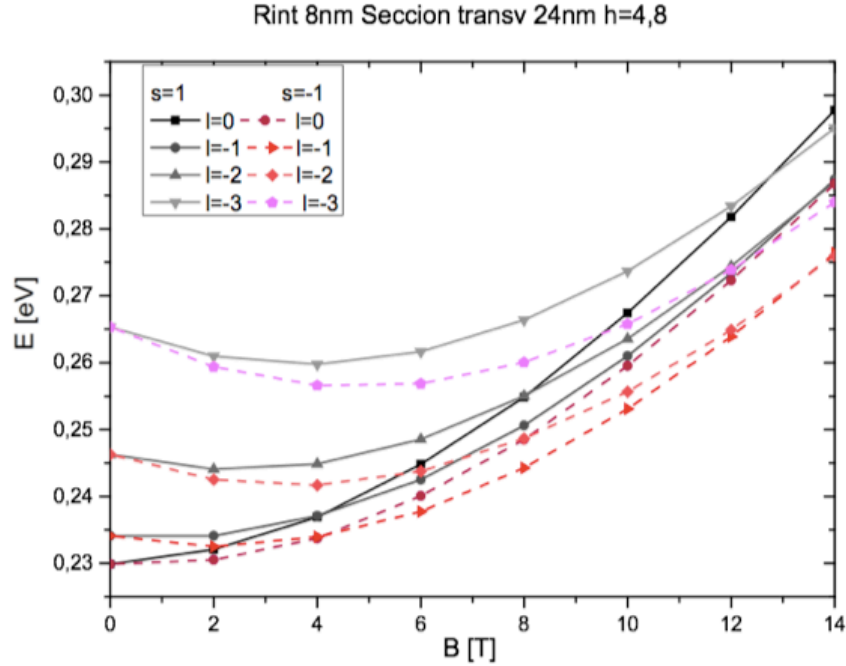
Figura 3.6: Estados confinados para radio R_{int} = 8 nm, altura h = 4.8 nm y el espín s tiene valores s = 1 y s = -1 , s = \pm 1 se refiere a la orientación del espín del electrón a lo largo del eje z .
