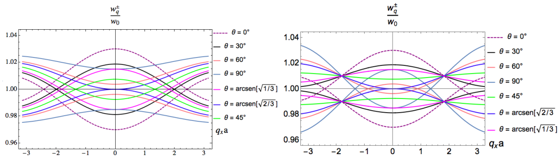
Figura 4.18: Dispersión colectiva de plasmones a lo largo de K'\Gamma K ( q_y a = 0 ) para diferentes orientaciones \theta de los dipolos. Izq. armchair ( \varphi = 0 ). Der. zigzag ( \varphi = 90 ).
