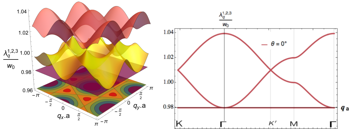
Figura 4.7: Izq: Dispersión colectiva de plasmones \theta = 0^\circ . Der: Estructura de bandas a lo largo de los puntos de alta simetría K-\Gamma-K'-M-\Gamma .
