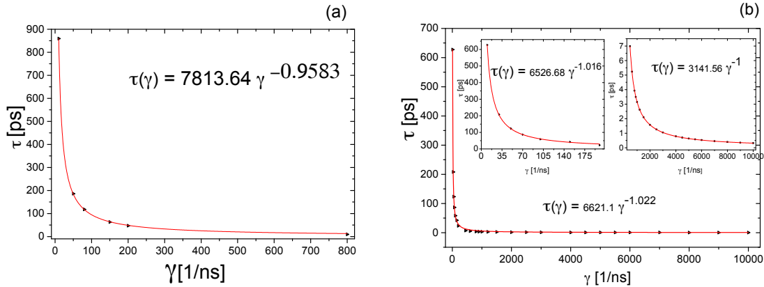
Figura 2.5: Aproximación de Weiss. Tiempos de relajación para diferentes valores de \gamma de una distribución de QD cónicos con radio (a) 4 nm y (b) 15 nm. Los recuadros b) muestran diferentes rangos de \gamma .
