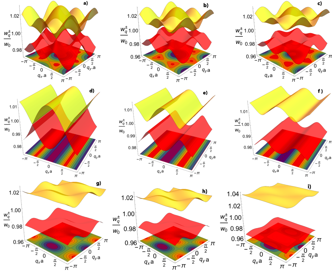
Figura 4.19: Dispersiones de plasmones colectivos de la ecuación (4.47) para \theta = 0 , a) d=0 , b) d=0.004 y c) d = 0.01 ; \theta = \arcsen[1/\sqrt{3}] , d) d=0 , e) d=0.004 , f) d=0.01 ; \theta = \pi/2 y g) d=0 , h) d=0.004 , i) d=0.06 .
