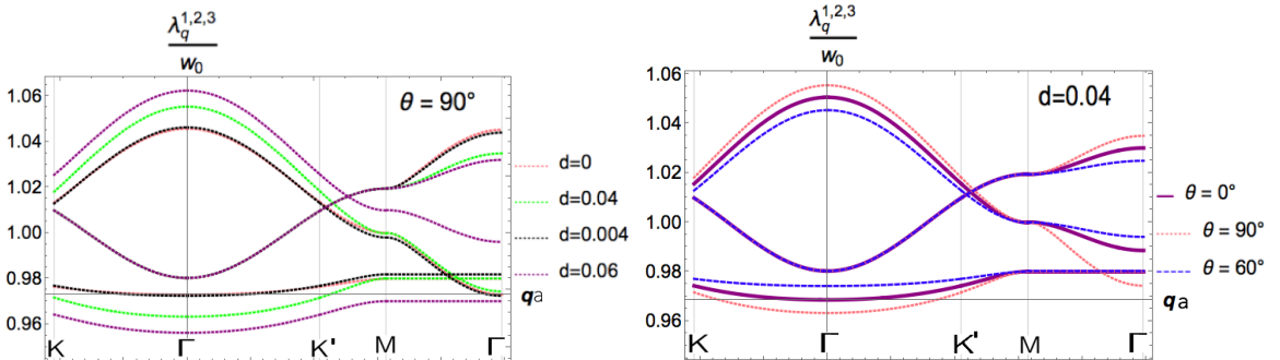
Figura 4.14: Dispersión colectiva de la trayectoria K - \Gamma - K' - M - \Gamma : Izq. \theta = 90 . Der. en función del parámetro d y \theta = 0, 90^\circ y 60^\circ
