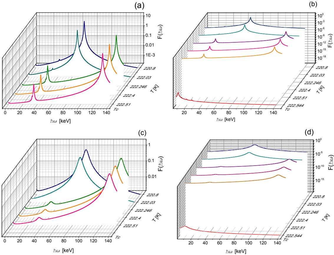
Figura 2.4: Función de pérdida de energía de una distribución de QDs cónicos con un radio de 15 nm, en la aproximación de Bragg-Williams. (a) - (b) \gamma = 500 \text{ ns}^{-1} , (c) - (d) \gamma = 4500 \text{ ns}^{-1} . b) y d) incluyen la función de pérdida para temperaturas cercanas a T_C . Observe las diferentes escalas.
