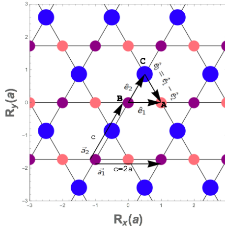
Figura 4.12: Red Kagomé infinita con inversión de simetría rota. Las sub-redes A,B tienen radio r_1 , y la sub-red C tiene radio r_2 .
