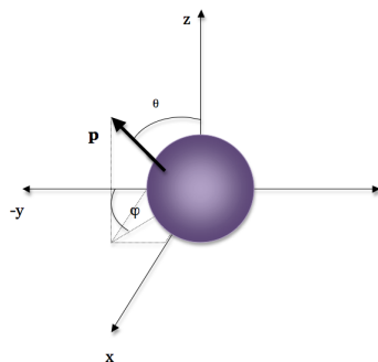
Figura 4.1: Orientaciones de los dipolos en coordenadas esféricas, mostrando los ángulos \theta y \varphi .
