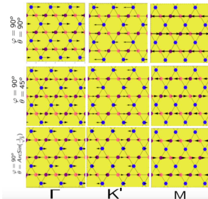
Figura 4.11: Distribución de fase de los dipolos para los modos \varphi = 90^\circ y (\theta = 90^\circ, \theta = 45^\circ, \theta = \text{Arcos}[1/\sqrt{3}]) .
