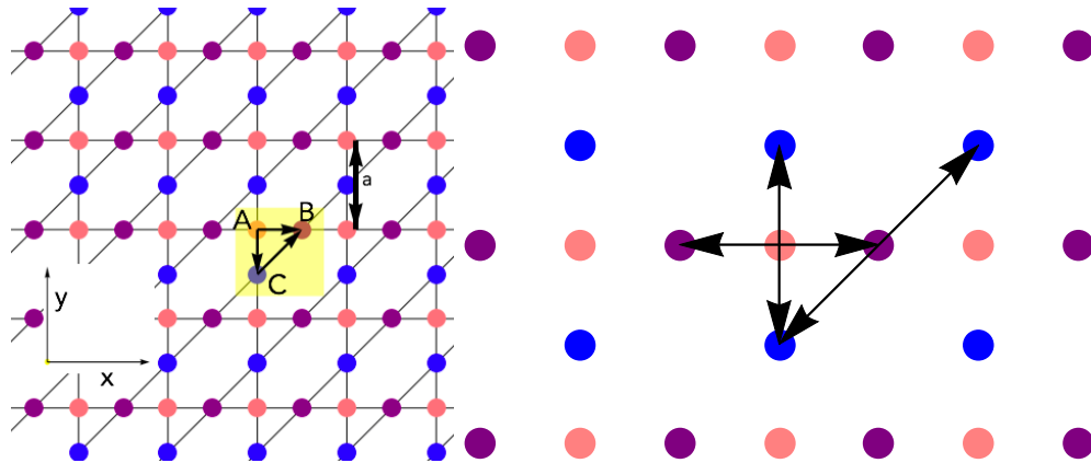
Figura A.1: Red Lieb (equivalente topológico de la red Kagomé) con constante de red a , que consta de tres subredes, etiquetadas como A, B y C, conectadas por los vectores entre vecinos más cercanos: \hat{e}_1 = \frac{a}{2}(1, 0) , \hat{e}_2 = \frac{a}{2}(0, -1) y \hat{e}_3 = \hat{e}_1 - \hat{e}_2 = \frac{a}{2}(1, 1) en cada celda unitaria (amarillo). Se puede notar que los vecinos más cercanos de cada partícula pertenecen a las otras subredes.
