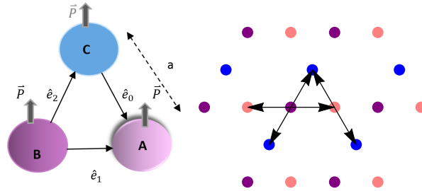
Figura 4.4: Representación de la interacción de partículas en la celda unidad. Se puede notar que los vecinos más cercanos de cada partícula pertenecen a las otras sub-redes.
