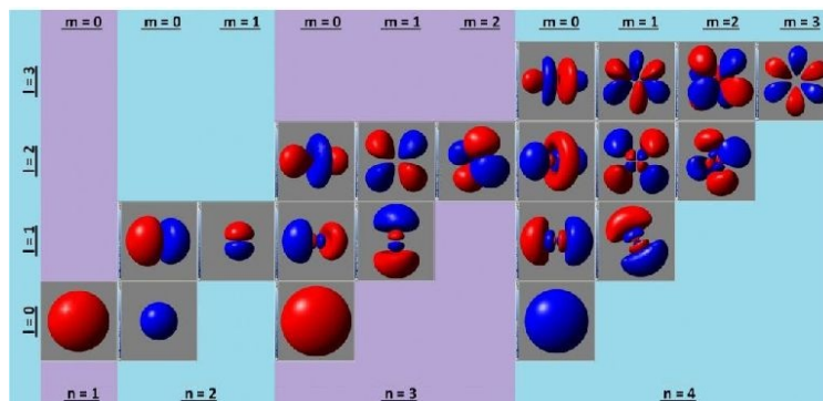
Figura 1.4: Representación de los orbitales electrónicos que surgen de la ecuación de Schrödinger para átomos con un solo electrón. Las funciones de onda son dependientes de los valores (n, l, m) , y muestran la región espacial con mayor probabilidad de encontrar un electrón. Las regiones azul/roja tienen diferente fase de función de onda.
