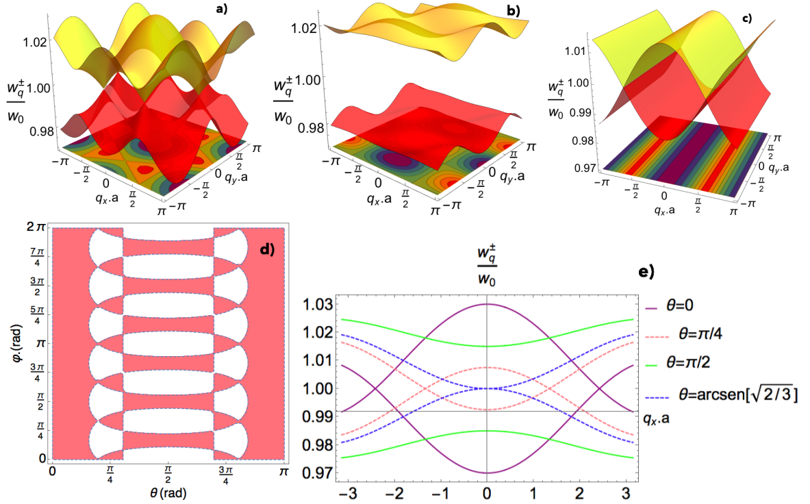
Figura 4.17: a), b) y c) Dispersión colectiva de plasmones de la ecuación (4.46). d) Representa el diagrama de fase para los ángulos (\theta, \varphi) de la dispersión de plasmones. La región rosa indica una región sin brecha entre las bandas, y la blanca indica la región con gap entre las dos bandas de dispersión de CPs. e) Dispersión colectiva de plasmones a lo largo de K'\Gamma K ( q_y a = 0 ) para diferentes orientaciones \theta de los dipolos. Para las figuras a)-d) \varphi = 0^\circ , y \Omega/\omega_0 = 0.01 .
