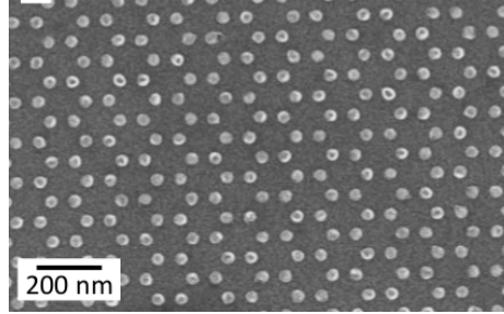
Figura 1.3: Imagen de microscopio electrónico de barrido (SEM), de un metamaterial plasmónico de un arreglo panal de nanodiscos de oro (Diego Scarabelli et al. ) [19].
