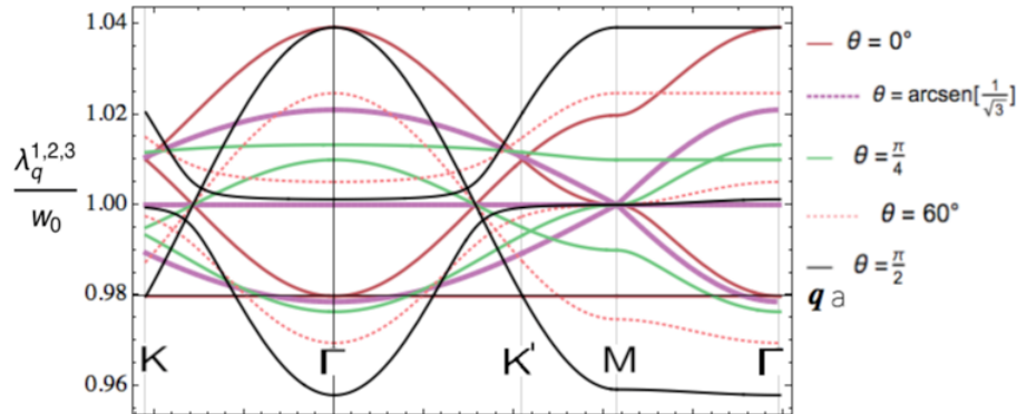
Figura 4.9: Dispersión colectiva de plasmones a lo largo de \text{K}-\Gamma-\text{K}'-\text{M}-\Gamma para el modo 0 < \theta \leq \pi/2 , y \varphi = \frac{\pi}{2} .
