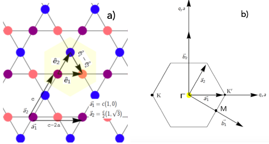
Figura 4.3: a) Estructura de Kagomé con constante de red a , que consta de tres sub-redes, etiquetadas como A, B y C, conectadas por los vectores entre vecinos más cercanos: \hat{e}_1 = a(1,0) , \hat{e}_2 = \frac{a}{2}(1, \sqrt{3}) y \hat{e}_0 = \hat{e}_1 - \hat{e}_2 = \frac{a}{2}(1, -\sqrt{3}) en cada celda Wigner-Seitz (amarillo). b) Primera zona de Brillouin (ZB) en el espacio recíproco con los vectores primitivos \mathbf{b}_1 y \mathbf{b}_2 .
