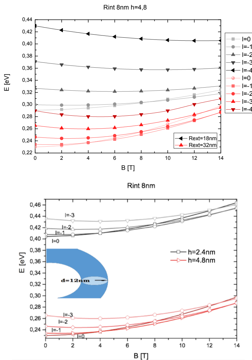
Figura 3.5: Superior. Estados confinados para R_{ext} = 18 nm y R_{ext} = 32 nm. Altura del eje menor de la sección elíptica ( h = 4.8 nm). Inferior. Estados confinados para R_{ext} = 32 nm. Altura del eje menor de la sección elíptica ( h = 2.4 nm y h = 4.8 nm).
