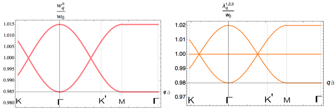
Figura 4.22: Estructura de bandas: Izq. Honeycomb . Der. Kagomé .
