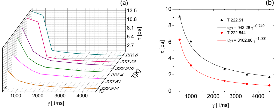
Figura 2.7: Aproximación de Bragg-Williams. Una distribución de QDs cónicos con un radio de 15 nm, tiempos de relajación a) para diferentes valores de \gamma y temperatura, b) dos valores de temperatura muestran dependencia de ley de potencia diferente.
