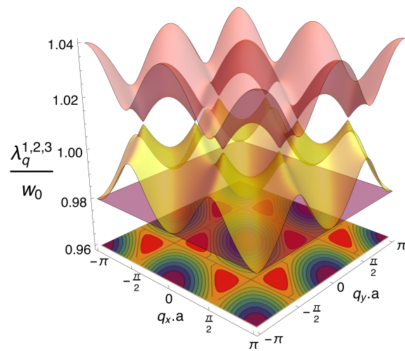
Figura A.2: Dispersión colectiva de plasmones \theta = 0^\circ y \varphi = 0^\circ .
