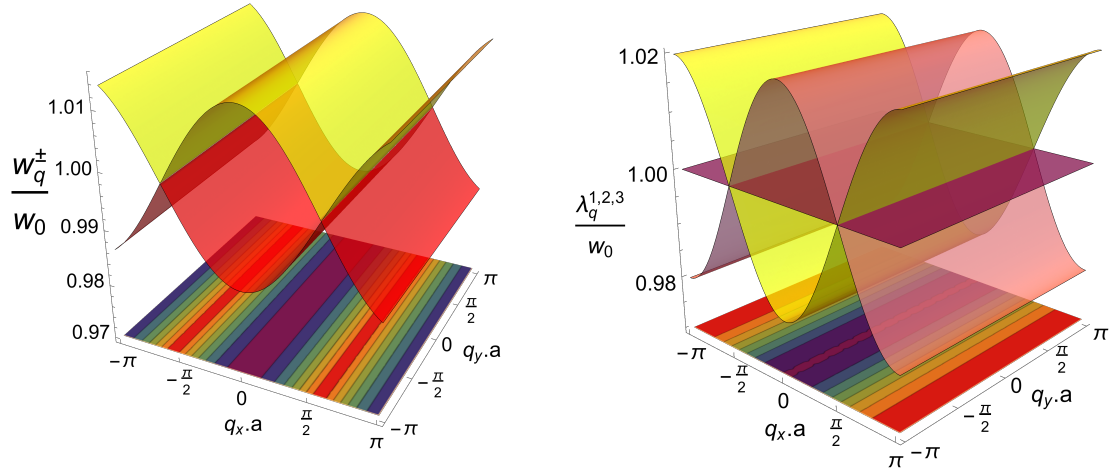
Figura 4.21: CPs para \varphi = 0 de Honeycomb y Kagomé plasmónico con \theta = \arcsen[\sqrt{1/3}] . Der. \theta = \arcsen(2/3) .
