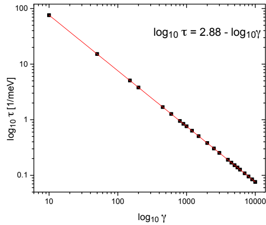
Figura 2.6: Tiempo de relajación para diferentes valores de \gamma de una distribución de puntos cuánticos cónicos de radio 15nm. Aproximación Weiss.
