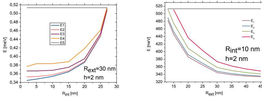
Figura 3.2: Izq. Estados confinados del anillo cuántico con radio externo 30 nm fijo, y para distintos radios internos. Der. Estados confinados para distintos radios externos y radio interno fijo 10 nm.
