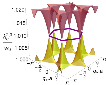
Figura 4.8: Dispersión de los modos colectivos cerca de los puntos K . Se puede notar el comportamiento lineal de las bandas cerca de estos puntos de alta simetría.
