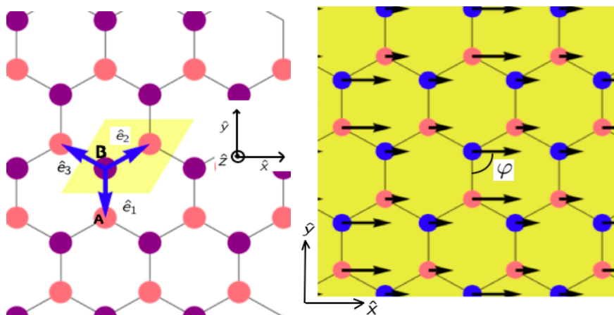
Figura 4.16: Izq. Estructura honeycomb con constante de red a , que consta de dos sub-redes, etiquetadas como A y B , conectadas en cada celda primitiva (amarillo) por los vectores entre vecinos más cercanos: \hat{e}_1 = a(0, -1) , \hat{e}_2 = \frac{a}{2}(\sqrt{3}, 1) y \hat{e}_3 = \frac{a}{2}(-\sqrt{3}, 1) . Der. Red honeycomb infinita de nanopartículas metálicas con momentos dipolares oscilatorios (Se muestra el ángulo \varphi en el plano).
