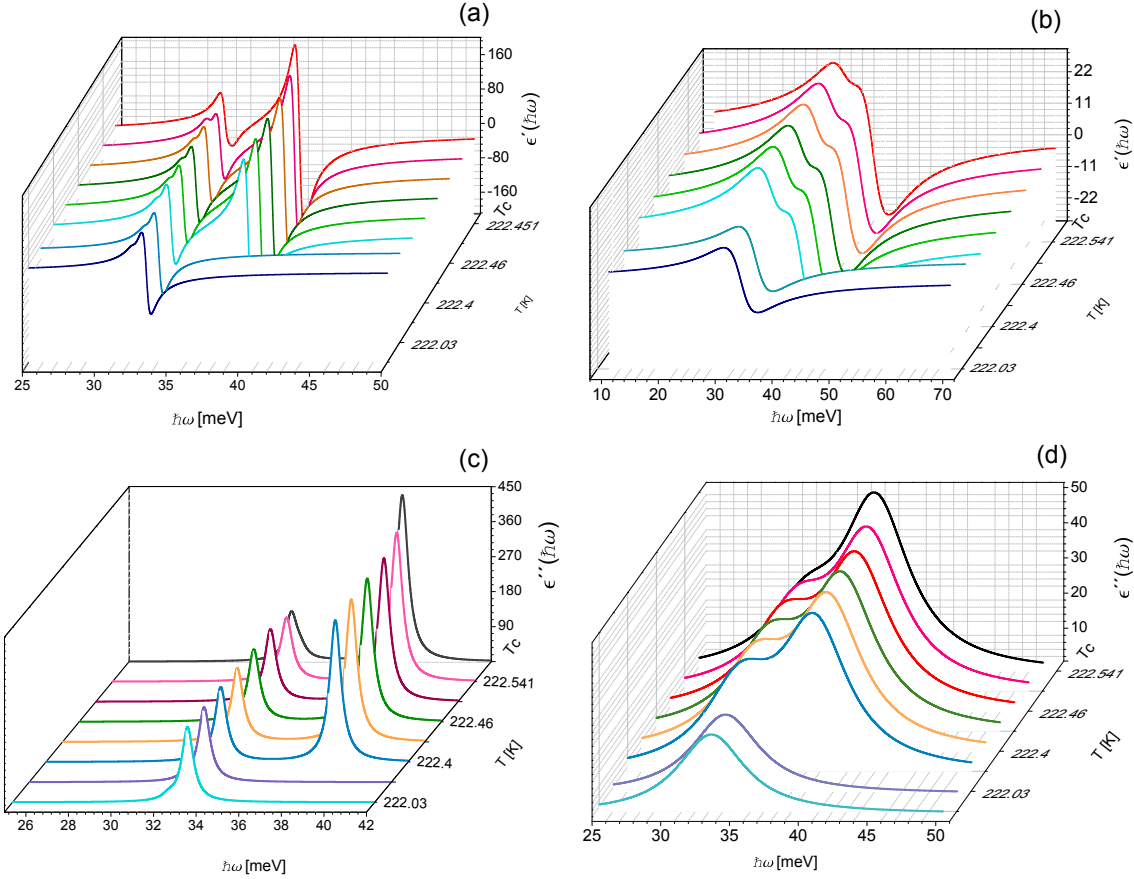
Figura 2.3: El comportamiento real (a)-(b), y (c)-(d) parte imaginaria de la función dieléctrica en función de la frecuencia, para una distribución de QD cónicos en la aproximación de Bragg-Williams. Esta aproximación predice tres bandas de resonancia diferentes, aunque los anchos dependen del parámetro de amortiguamiento \gamma . (a) - (c) \gamma = 500 \text{ ns}^{-1} , (b) - (d) \gamma = 4500 \text{ ns}^{-1} .
