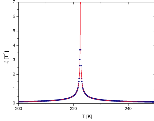
Figura 2.2: Correlación en función de la temperatura de puntos cuánticos cónicos con radio 15nm bajo acción de campos eléctrico E_{mol} = 1 meV/nm y E_{ext} = 1 meV/nm, T_C = 222.55 K.
