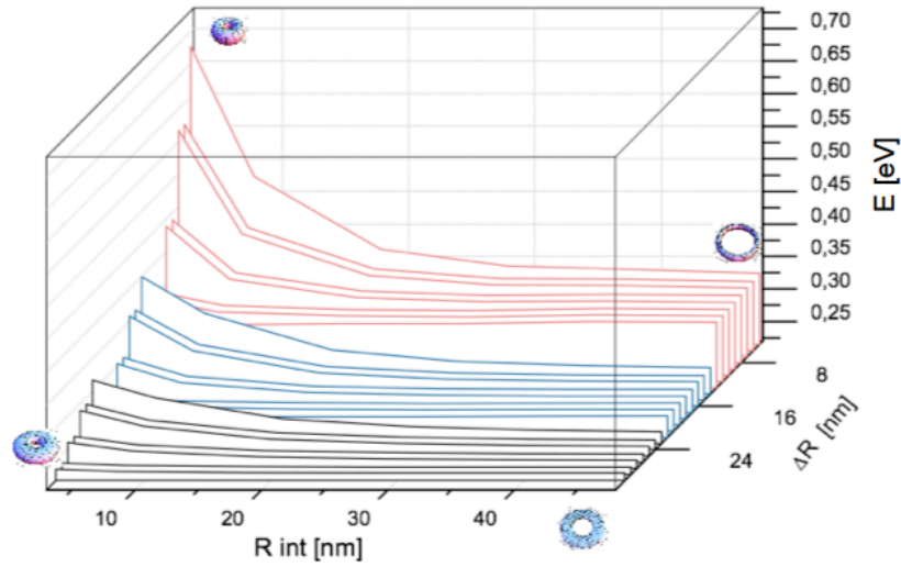
Figura 3.4: Estados confinados de radio externo y radio interno.
