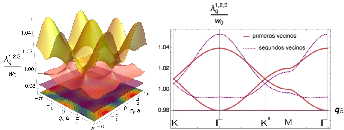
Figura 4.15: Izq. Dispersión colectiva incluyendo interacciones con segundos vecinos para polarización de PSL \theta = 0 y \varphi = 0 . Der. Bandas de dispersión colectiva a lo largo de K - \Gamma - K' - M - \Gamma' . Curvas rosas indican la dispersión que incluye solo interacciones de primeros vecinos, curvas violetas incluyen interacciones de primeros más segundos vecinos.
