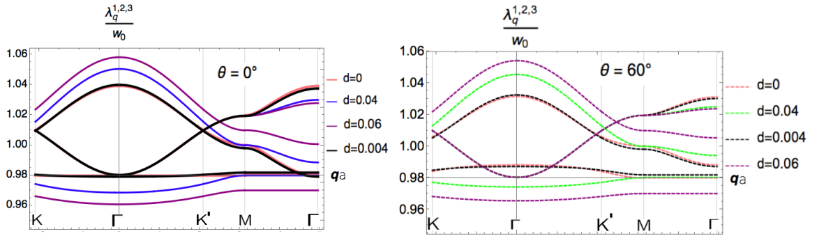
Figura 4.13: Dispersión colectiva de la trayectoria K - \Gamma - K' - M - \Gamma en función del parámetro d . Izq. \theta = 0 . Der. \theta = 60^\circ
