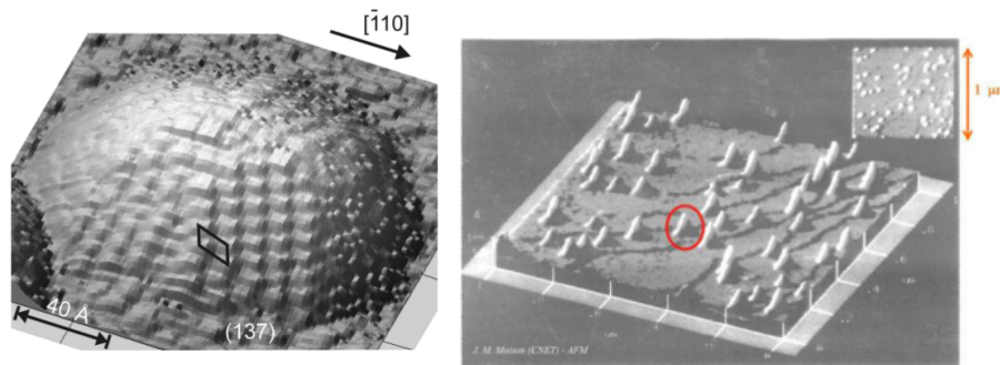
Figura 1.1: Izq. Imagen tridimensional de microscopio de efecto túnel (STM) de un punto cuántico sin cubrir de InAs crecido sobre GaAs (001) (Instituto Fritz-Haber, Berlin [1]). Der. Imagen obtenida por microscopio de fuerza atómica (AFM) de QDs de InAs/GaAs autoensamblados [2].
