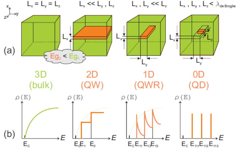
Figura 1.5: (a) Comparación esquemática de las dimensiones típicas de material en bulto (bulk), pozo (QW), hilo (QWR) y punto cuántico (QD). El confinamiento se realiza insertando un semiconductor en otro con mayor ancho de banda. (b) Las densidades de estados correspondientes a las estructuras que se muestran en (a). Las energías están indexadas por los números cuánticos correspondientes n_1, n_2, n_3 .
