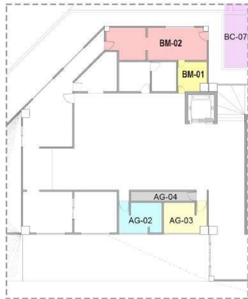
Planta arquitectónica baja
