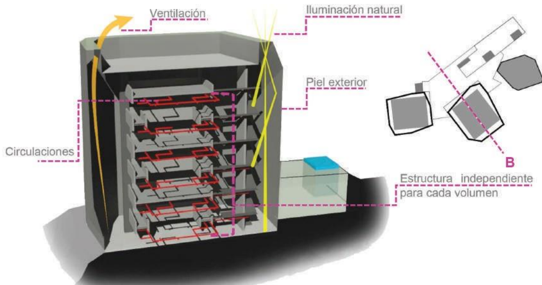
Esquema 12. Parque Biblioteca España, corte B, diseño interior-Biblioteca. Fuente: Internet.
