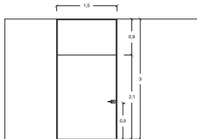
PUERTA TIPO 2
