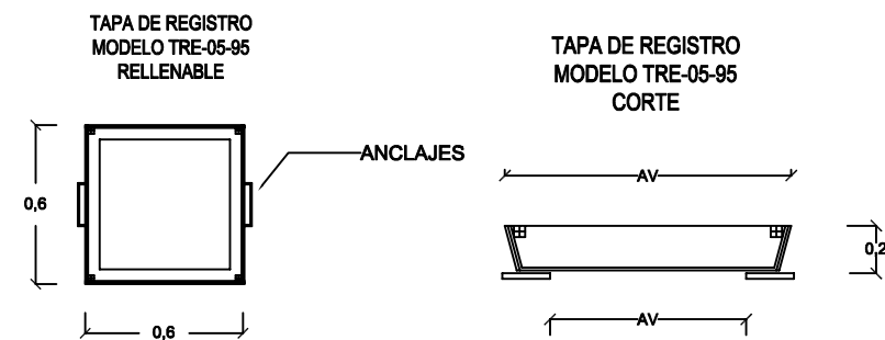
DETALLE REGISTRO
