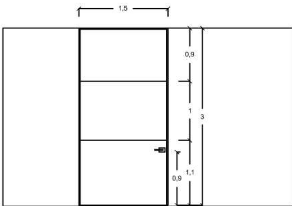
PUERTA TIPO 1
