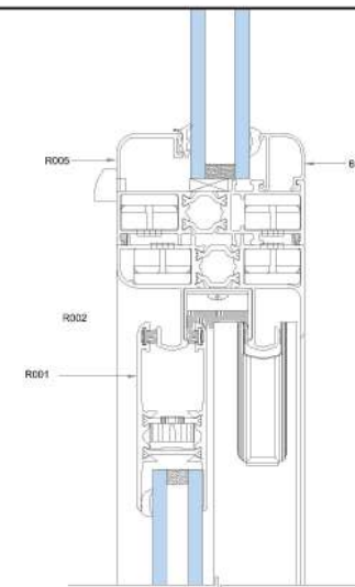
DETALLE 6
