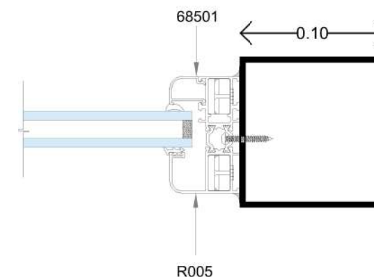
DETALLE 7
