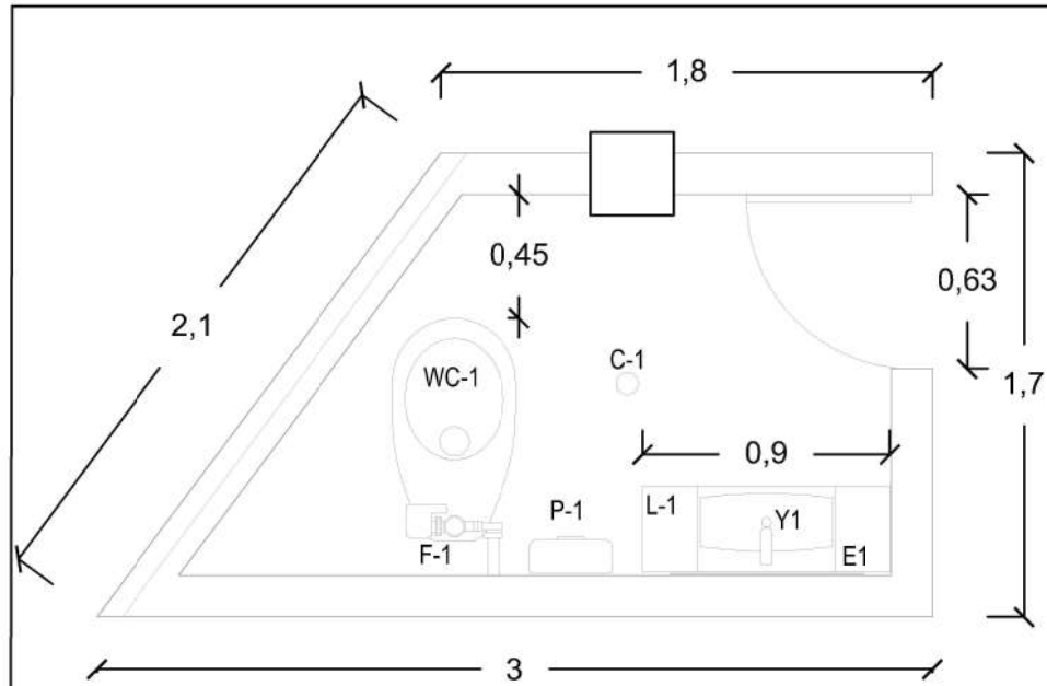
PLANTA ARQUITECTONICA BAÑOS LOCAL 1 ESC. 1:30
