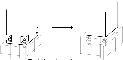
Detalle de columna
