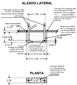
MUERTO DE CONCRETO DETALLE 01 ESCALA 1:100 COTAS: MTS
