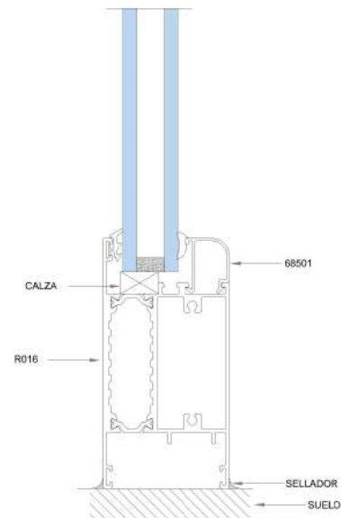
DETALLE 2 DETALLE DE UNIÓN INFERIOR DE PERFIL FIJO A PISO
