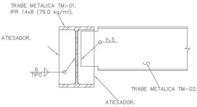
CONEXION CON-02
