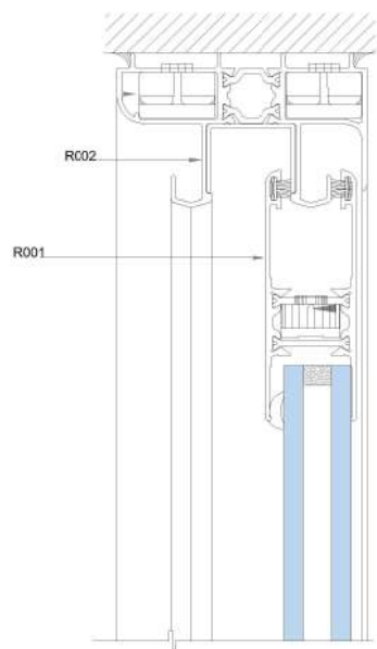
DETALLE 3 DETALLE DE DE PERFIL SUPERIOR DE PUERTA CORREDIZA
