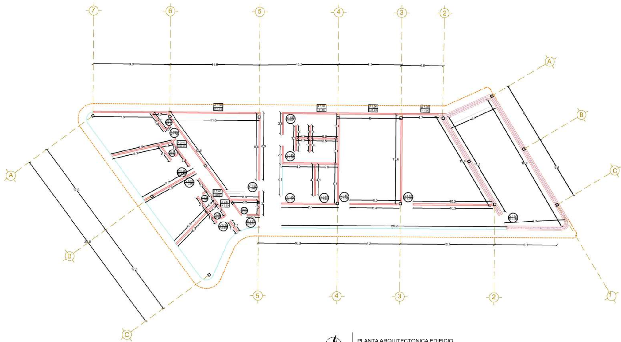
PLANTA ARQUITECTONICA EDIFICIO NPT +/- 0.00
