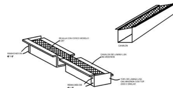
DETALLE DE TAPA DE CANALON PRESPECTIVA
