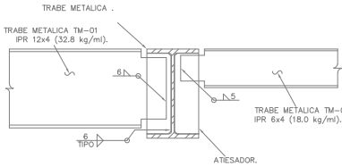
CONEXION CON-03
