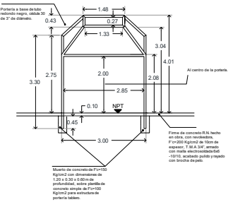
ALZADO FRONTAL DE PORTERÍA ESCALA 1:100 COTAS: MTS
