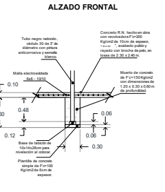
MUERTO DE CONCRETO DETALLE 02 ESCALA 1:50 COTAS: MTS
