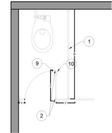
DETALLE MAMPARA
