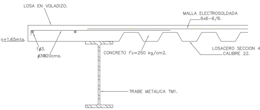
DET-01 DETALLE DE BORDE DE LOSA (sera curvo en el volado)
