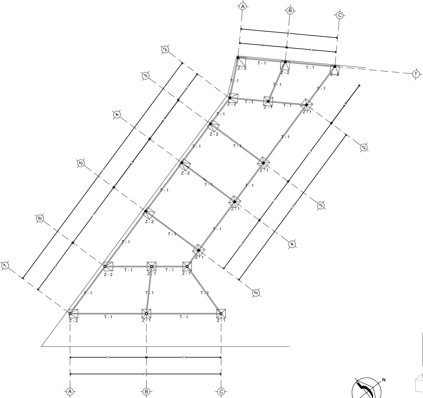
PLANTA DE CIMENTACIÓN
