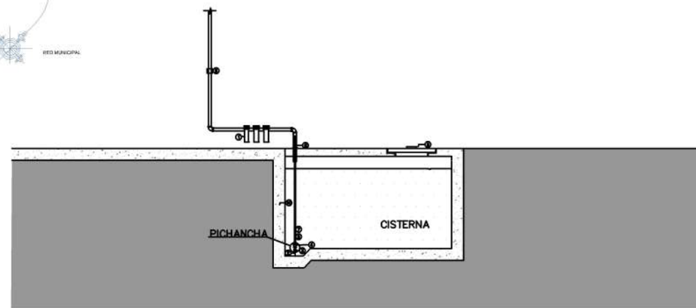
DETALLE 1 SISTEMA DE CAPTACION PLUVIAL
