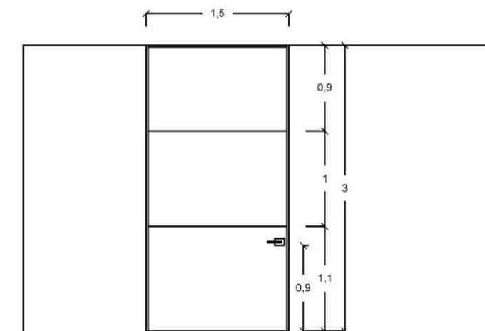
PUERTA TIPO 1
