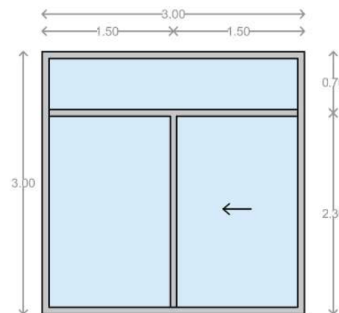
CANCEL TIPO 04 ESC 1: 60
