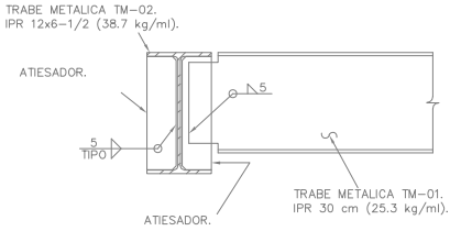
CONEXION CON-01
