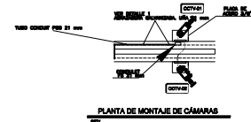
PLANTA DE MONTAJE DE CÁMARAS
