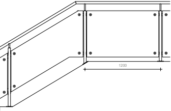
Detalle para elementos en rampa
