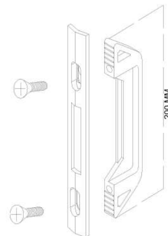
FN-604C ENGANCHE DE CIERRE (EXTERIOR)
