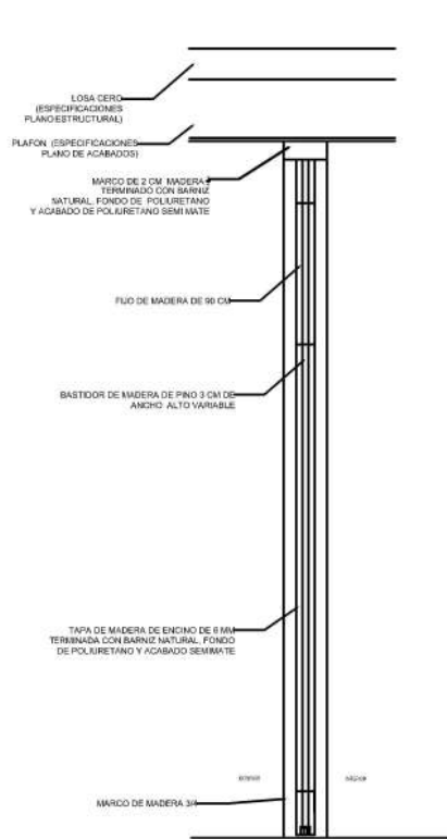
CORTE PUERTA
