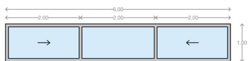
VENTANA TIPO 04 ESC 1: 60
