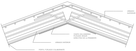
DET-02 DETALLE DE INCLINACION DE LOSA
