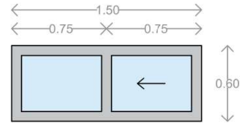
VENTANA TIPO 01 ESC 1: 30
