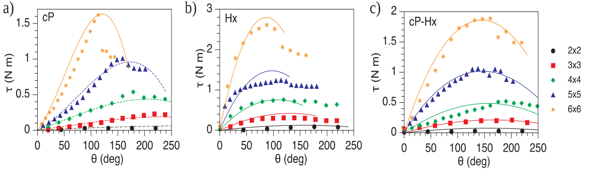
Figura 2.18: (a-c) Resistencia a la torsión \tau opuesta por los tres tipos de estructuras a la deformación angular \theta . Los puntos representan valores obtenidos experimentalmente para cada estructura, las líneas continuas muestran los resultados obtenidos de simulaciones numéricas.
