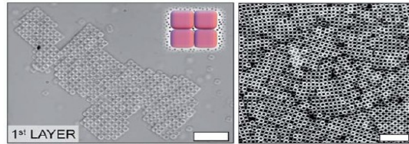
Figura 2.2: Autoensamblaje en cristales cúbicos de hematita. La presión osmótica ejercida por el polímero favorece el contacto entre los cristales cúbicos de hematita. Imágenes obtenidas de [41].
