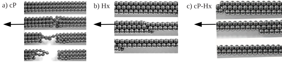
Figura 2.11: Proceso de deformación en magnetocristales sometidos a esfuerzos de tensión: a) cP, b) Hx y c) estructuras cP-Hx.
