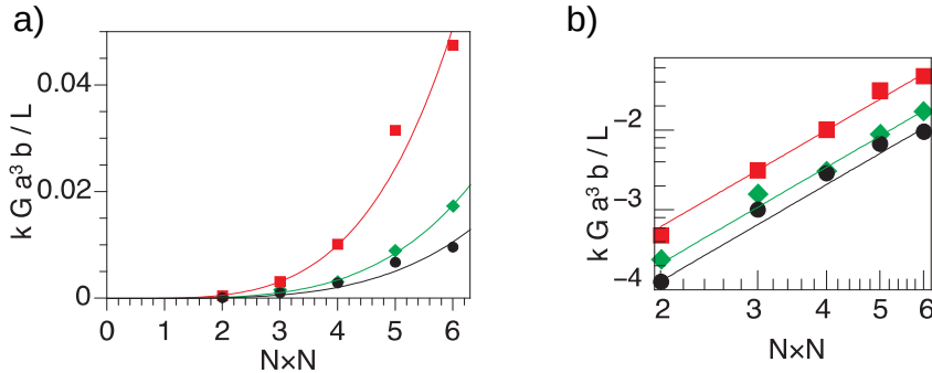
Figura 2.19: a) s_3 como función de las dimensiones del cristal N \times N para Hx (cuadros rojos), cP (puntos negros) y cristales híbridos (rombos verdes). b) Gráfico log s_3 vs log N el cual indica una dependencia con N^4 , las líneas continuas indican las curvas ajustadas.
