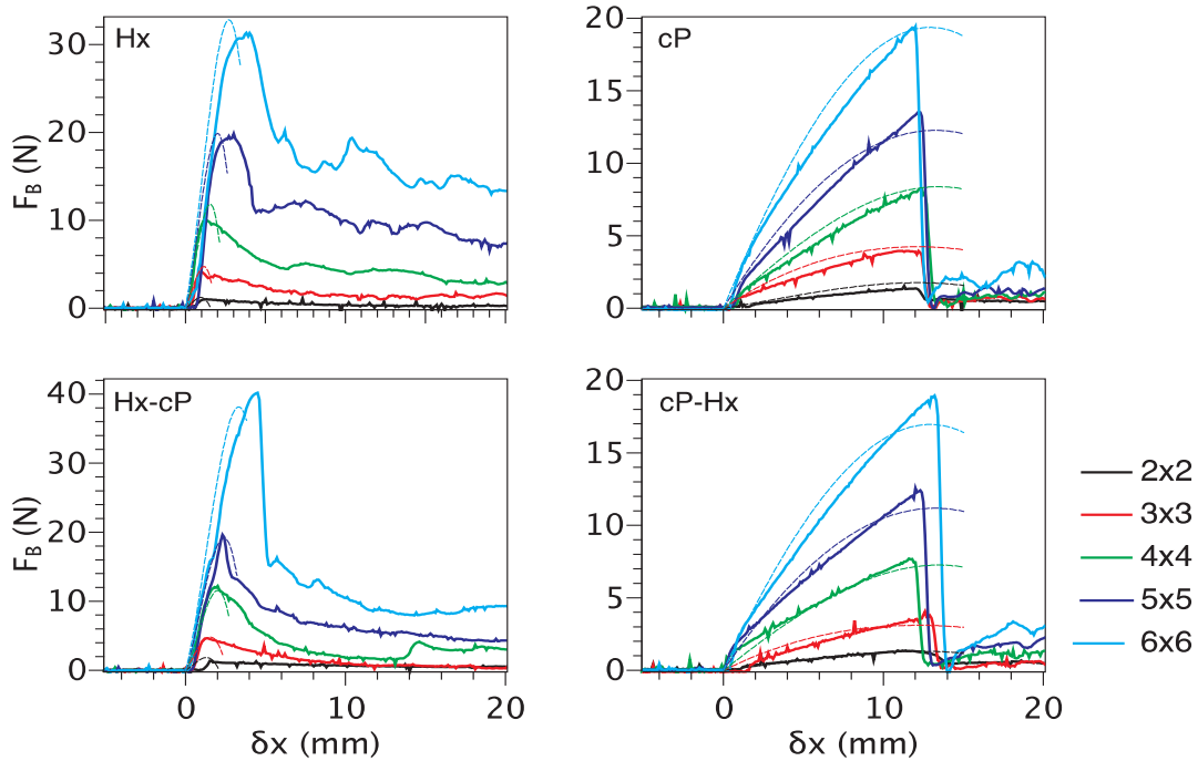
Figura 2.15: Fuerza de flexión experimental F_B requerida para producir una deformación perpendicular \delta x en los ensambles Hx, cP y cP-Hx de diferente tamaño (líneas sólidas). El gráfico Hx-cP, indica que la fuerza en la estructura híbrida se aplica sobre el plano con configuración Hx, mientras que el cP-Hx indica que la fuerza se aplica sobre el plano cP de la estructura. Las líneas a trazos corresponden con las simulaciones REM. Las curvas con \delta x < 0 representan valores de fuerza medidos antes de aplicar el esfuerzo sobre la estructura.
