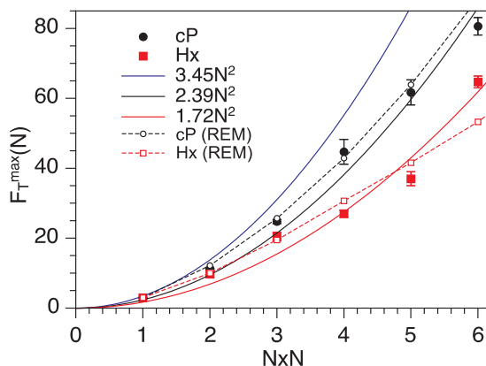
Figura 2.13: Fuerza máxima de ruptura F_T^{max} de magnetocristales sometidos a fuerza de tensión como función de las dimensiones del cristal N \times N (puntos sólidos). Las curvas continuas corresponden a F_T^{max} \propto N^2 y las curvas a trazos con las simulaciones de minimización de energía.
