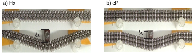
Figura 2.14: Montaje experimental: a) Magnetocrystal Hx y b)cP, sometidos a esfuerzo de flexión. Note que la estructura Hx se rompe (forma de V) mientras que la matriz cP se dobla, en ambos se mide la deformación perpendicular \delta x .
