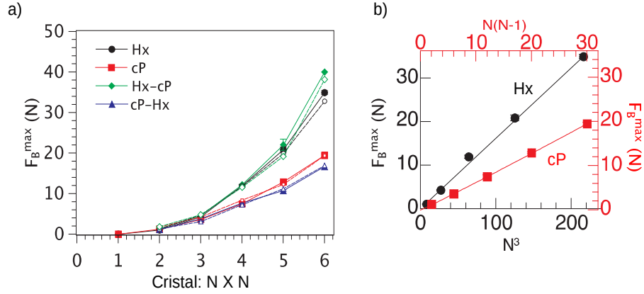
Figura 2.16: Fuerza máxima de flexión F_B^{max} para magnetocristales cP y Hx como función del tamaño del cristal N \times N , experimentos (puntos sólidos) y simulaciones (puntos abiertos). A la derecha se muestra que F_B^{max} \propto N^3 para la estructura hexagonal y F_B^{max} \propto N(N-1) para la estructura cP.
