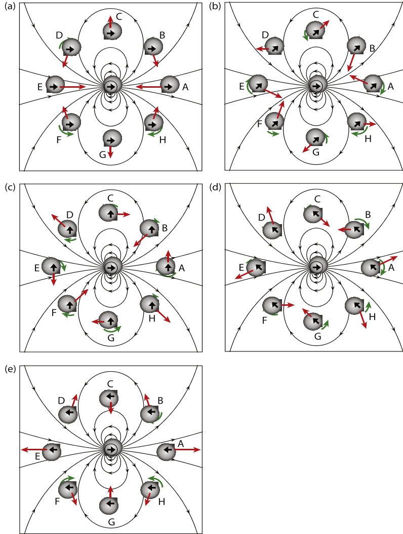
Figura A.2: Líneas de campo producidas por una esfera uniformemente magnetizada con un momento magnético total \vec{m}_1 en el centro de cada panel y las fuerzas magnéticas resultantes y torcas sobre una esfera uniformemente magnetizada de momento magnético total \vec{m}_2 , en varias posiciones y orientaciones. Se muestran las figuras para \vec{m}_2 y \vec{m}_1 en diferentes configuraciones para \beta a) 0, b) \pi/4 , c) \pi/2 , d) 3\pi/4 y e) \pi . Para cada panel hay 8 posiciones de la esfera 2, representados por A-H, distribuidos uniformemente alrededor de un círculo centrado en la esfera 1. Los vectores de fuerza se presentan con longitud proporcional a la magnitud de la fuerza. Las torcas se muestran por medio de arcos con longitud proporcional a la magnitud de la torca y sin arco cuando la torca es cero. La dirección del momento magnético se indica con flechas negras. Imagen obtenida por medio del software Magphyx [29].
