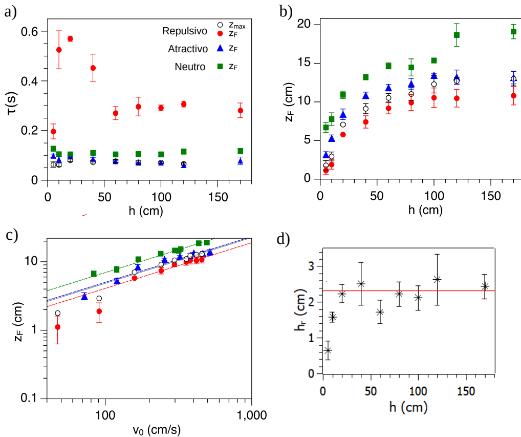
Figura 3.14: Resultados experimentales. a) Tiempo de penetración \tau vs altura de impacto h para los tres tipos de proyectil. El tiempo máximo de penetración para el caso repulsivo se muestra con el símbolo \circ . El tiempo total de penetración para el caso repulsivo (puntos rojos) es mayor debido a los rebotes que presenta. Para los casos atractivo y neutro \tau es aproximadamente constante. b) Profundidad final de penetración como función de h para los tres proyectiles. c) Gráfico log-log para z_{max} vs v_0 para el caso repulsivo comparado con z_F para los tres proyectiles. La pendiente de las curvas es 1/3 . d) La altura promedio de rebote del proyectil negativo tiene un valor \sim 2.3 cm. La leyenda a colores de a) es válida en b) y c).
