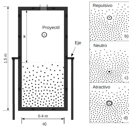
Figura 3.2: Esquema del montaje experimental. a) Celda Hele-Shaw parcialmente llena con discos magnéticos que se repelen entre sí. Un proyectil es lanzado desde la parte superior dentro de la celda, su penetración es filmada con cámara de alta velocidad. El proyectil puede experimentar interacción b) repulsiva, c) neutra o d) atractiva.
