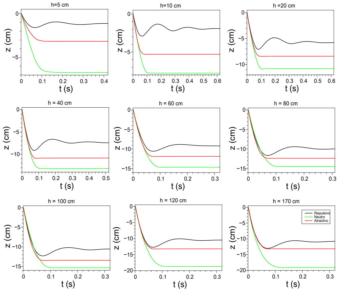
Figura 3.8: Comparación de z vs t de los tres tipos de proyectil impactando desde distintas alturas, el color de la curva representa el tipo de proyectil, la densidad de los proyectiles es \rho = 3.28 \text{ g/cm}^3 . La convención de colores es: negro-repulsivo, verde-neutro y rojo-atractivo.
