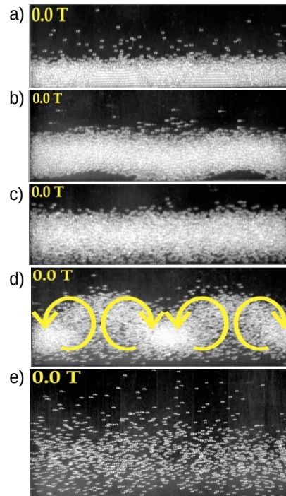
Figura 4.2: Se muestran los regímenes que exhibe un sistema granular convencional en presencia de gravedad. a) rebote, b) ondulaciones, c) efecto leidenfrost granular, d) rollos de convección y e) gas granular. Figura tomada de [7].
