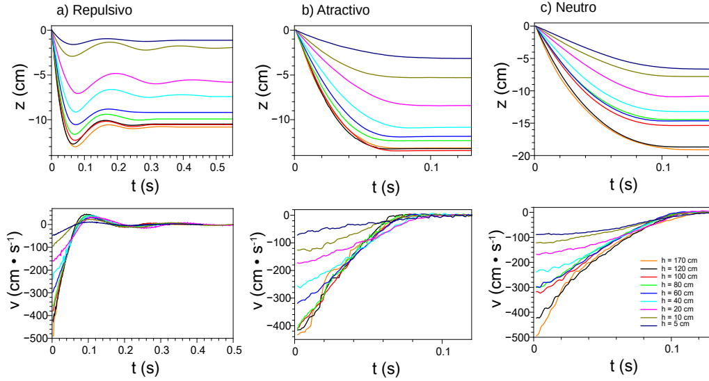
Figura 3.6: Dinámica de penetración experimental para interacciones a) repulsiva, b) atractiva y c) neutra con proyectiles ( \rho = 3.28 \text{ g/cm}^3 ) penetrando desde diferentes alturas h , z = 0 corresponde a la superficie de la cama granular. La máxima profundidad se alcanza aproximadamente a 0.1 s para los tres casos. El caso repulsivo se caracteriza por oscilaciones en la dinámica de penetración, con velocidades positivas correspondientes al rebote del proyectil. Note que el proyectil neutro penetra más profundo en los tres casos.
