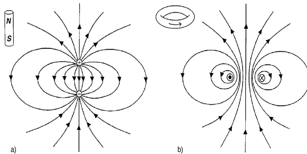
Figura 1.3: Dipolos magnéticos: a) modelo de carga magnética y campo \vec{H} ; y b) modelo de circuito de corriente y campo \vec{B} .
