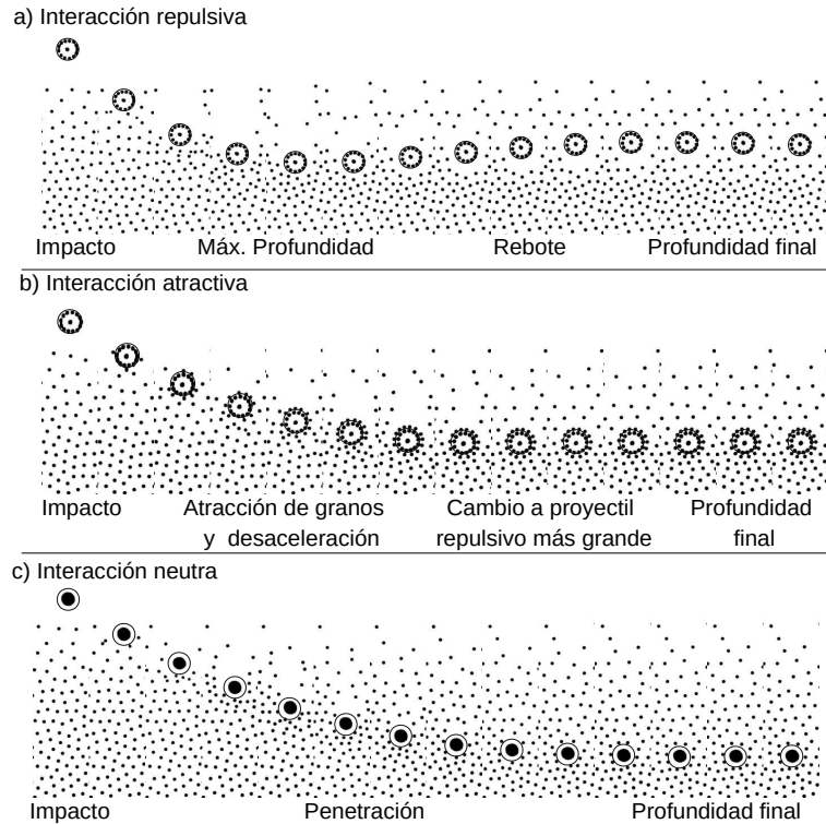
Figura 3.3: Instantáneas obtenidas de los videos de experimentos para impactos con interacciones: a) repulsiva, b)atractiva y c)neutra. El proceso de impacto y penetración se puede dividir en diferentes etapas dependiendo de la interacción cama-proyectil.
