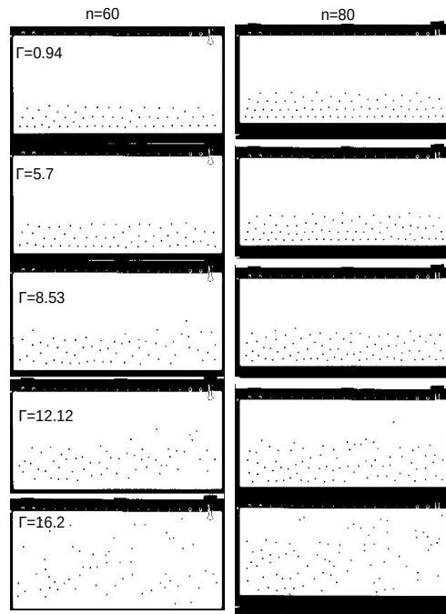
Figura 4.6: Se muestra la dinámica observada experimentalmente con una celda Hele Shaw vibrada verticalmente con granos magnéticos repulsivos en su interior, n representa el número de granos y \Gamma el parámetro de aceleración adimensional.
