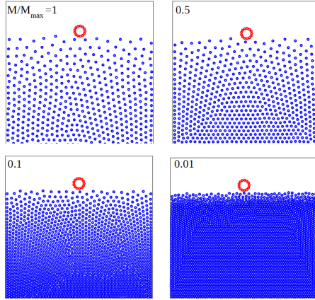
Figura 3.17: Usando dinámica molecular (MD) se construyen camas granulares con diferentes magnitudes de magnetización M/M_{max} . El caso M/M_{max} = 1 corresponde con el valor de la magnetización experimental.
