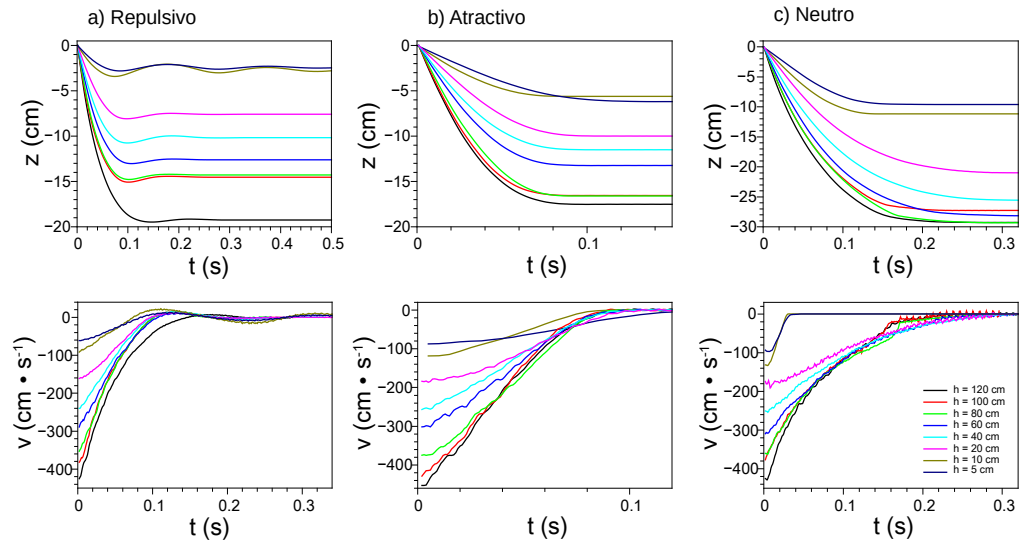
Figura 3.7: Dinámica de penetración para interacciones a)repulsiva, b)atractiva y c)neutra para experimentos con proyectiles ( \rho_2 = 5.2 \text{ g/cm}^3 ) penetrando desde diferentes alturas h .
