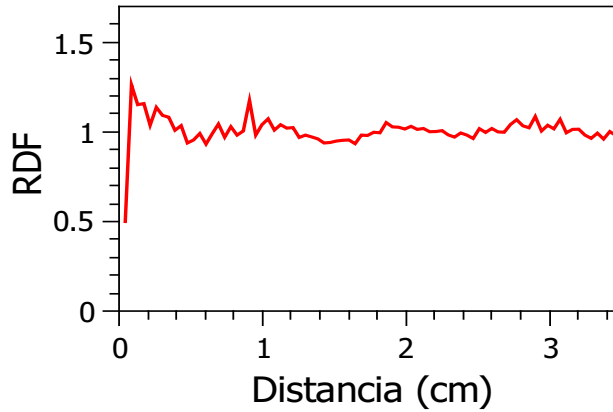
Figura 4.9: Función de distribución radial para un sistema con \Gamma = 16.2 y n = 120 . La curva indica una coexistencia de fases líquida y gaseosa.
