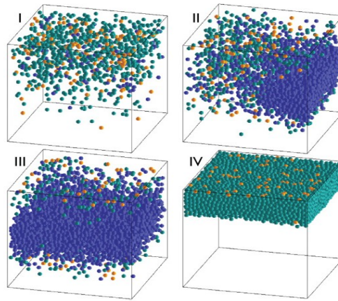
Figura 4.1: Se muestran los regímenes que exhibe un sistema granular convencional en microgravedad por medio de simulaciones con MD. I) estado gaseoso, II) aglomeración parcial, III) aglomeración completa y IV) aglomeración con rebote. Figura tomada de [95].
