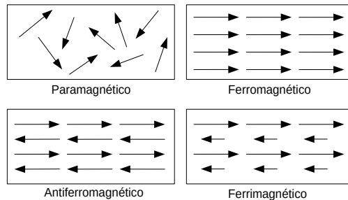
Figura 1.2: Clasificación de los materiales magnéticos. Las flechas representan los momentos dipolares magnéticos.
