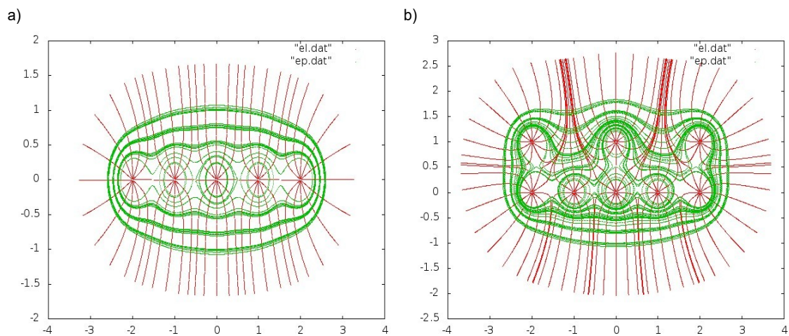
Figura 1.6: Líneas de campo magnéticas y curvas equipotenciales generadas por la interacción de imanes permanentes usando el modelo de carga. (a) Configuración para una capa con cinco imanes colineales y (b) ocho imanes con tendencia a la formación de doble capa.
