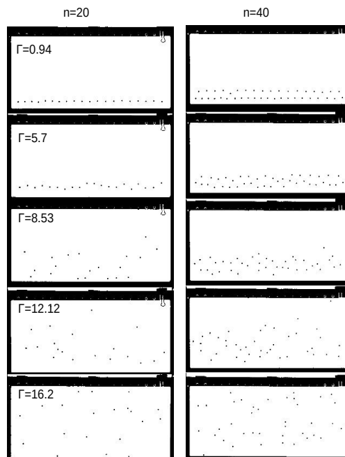
Figura 4.5: Se muestra la dinámica observada experimentalmente con una celda Hele Shaw vibrada verticalmente con granos magnéticos repulsivos en su interior, n representa el número de granos y \Gamma el parámetro de aceleración adimensional.
