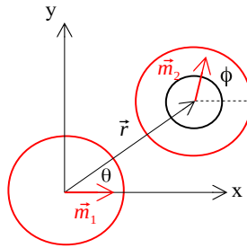
Figura A.1: Sistema de coordenadas polares para estudiar dos esferas magnéticas con igual radio. Una esfera con un momento magnético \vec{m}_1 se mantiene fija en el origen con su momento magnético en la dirección +x . Una segunda esfera con momento magnético \vec{m}_2 orientada un ángulo \phi se localiza en la posición \vec{r} con coordenadas polares (r, \theta) .
