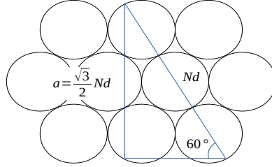
Figura 2.17: Geometría de la estructura hexagonal dos dimensional.
