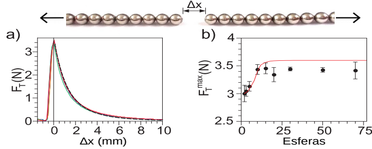
Figura 2.8: Fuerza de tensión requerida para fracturar una cadena: a) F_T vs \Delta x . Las líneas en color representan los datos experimentales y la línea negra a trazos representa F \propto \Delta x^{-4} . b) F_T^{max} como función del número de esferas magnéticas que conforman la cadena obtenida, experimentos (puntos negros) y simulaciones con dinámica molecular (línea roja).
