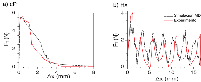
Figura 2.10: Fuerza de tensión F_T como función de la deformación \Delta x para una cadena 2D. Las líneas sólidas representan los experimentos y las líneas a trazos los resultados numéricos.
