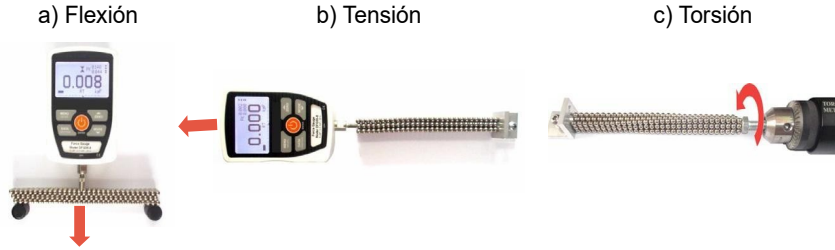
Figura 2.6: Arreglos experimentales usados para medir la respuesta mecánica de los cristales magnéticos ante la aplicación de: flexión, tensión y torsión. Las flechas en color rojo indican la dirección de la fuerza aplicada.
