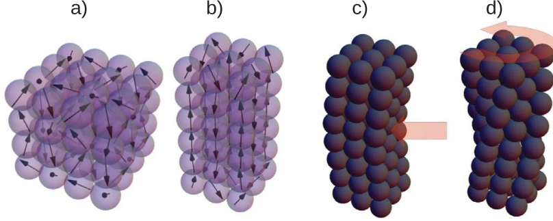
Figura 2.7: a) Orientaciones dipolares en una estructura cúbica de imanes esféricos permanentes. b) Si se aumenta el número de capas en una dirección, los dipolos se reorientan en una dirección. c-d) Ejemplos de estructuras cP construidas numéricamente y sometidas a flexión y torsión. Para simular la flexión, cada capa de la estructura se traslada lateralmente manteniendo las extremidades del cristal fijas. La torsión se simula girando cada capa del cristal (colaboración GrainsLab).
