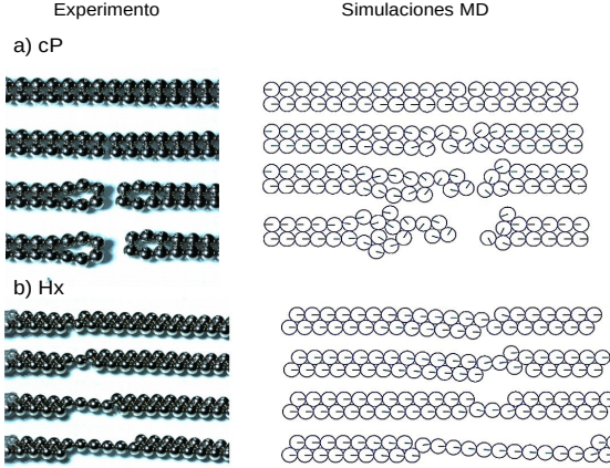
Figura 2.9: Cadenas 2D sometidas a esfuerzos de tensión: a) estructura cuadrada (cP) y b) estructura hexagonal (Hx). Los snapshots de la izquierda muestran el proceso de ruptura experimental.
