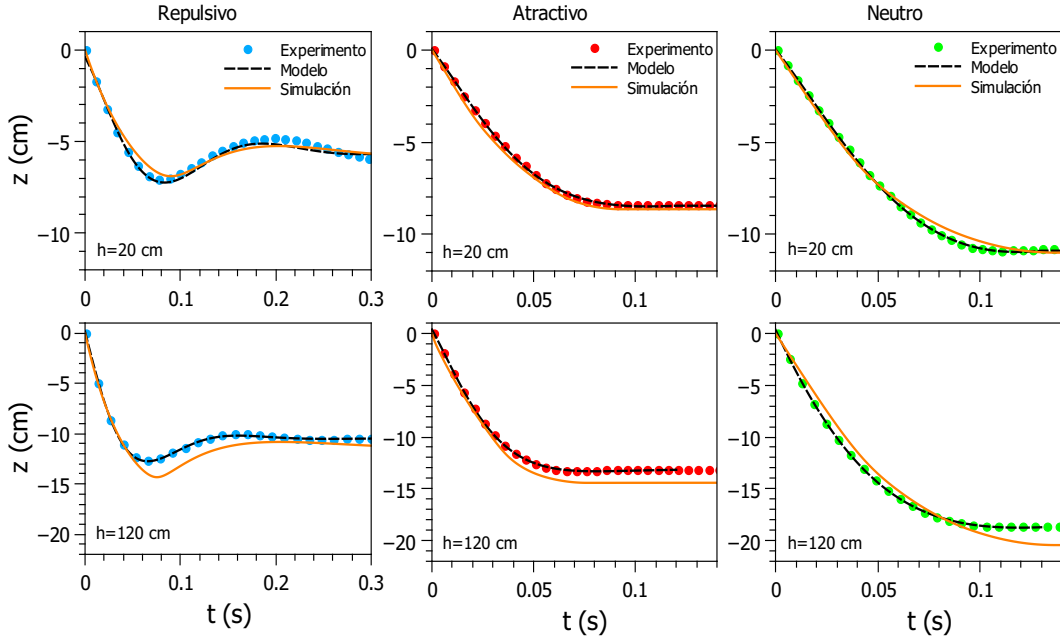
Figura 3.22: Dinámica de penetración de los tres proyectiles (repulsivo, atractivo y neutro) obtenida de los experimentos (puntos) y su comparación con el modelo (línea a trazos) y las simulaciones (línea sólida). Los resultados se muestran para h = 20 cm y h = 120 cm.
