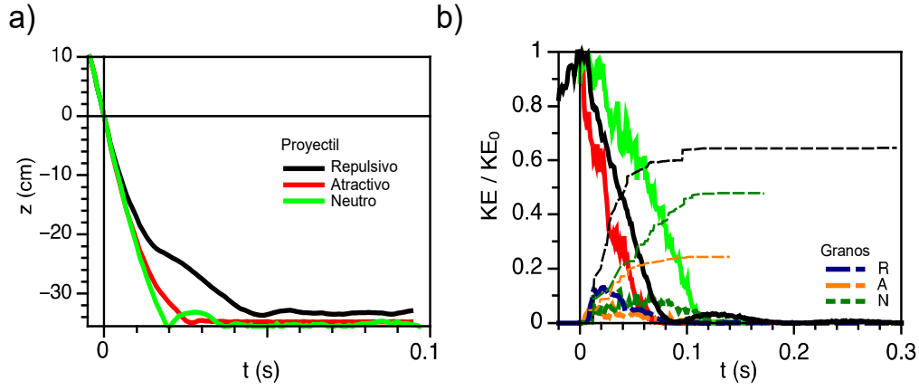
Figura 3.21: Resultados numéricos: a) Gráficos z vs t mostrando la dinámica de los tres proyectiles con partículas sin fricción considerando los casos repulsivo (curva negra), atractivo (curva roja) y neutro (curva verde). b) Se muestra la evolución temporal de la energía cinética (KE) para el proyectil (curvas sólidas: negro-repulsivo, rojo-atractivo, verde-neutro) y los granos de la cama granular (curvas a trazos: azul-repulsivo, anaranjado-atractivo, verde-neutro), la energía KE está normalizada con la energía de impacto del proyectil en t = 0 ( KE_0 ). La energía acumulada KE representa la suma de la energía cinética máxima de los granos que han interactuando con el proyectil desde t = 0 hasta un tiempo t , para los tres casos: repulsivo (línea a trazos negra), atractivo (línea a trazos verde) y neutro (línea a trazos anaranjada). La energía cinética de los granos es la suma de las energías de todos los granos a un tiempo t . En esta figura h = 20 cm. La energía acumulada representa la transferencia de energía relativa en el sistema. Por ejemplo, el proyectil repulsivo transfiere al sistema aproximadamente el 60% de su energía, esto indica que el 40% restante se disipa debido a la fricción con las paredes de la celda.
