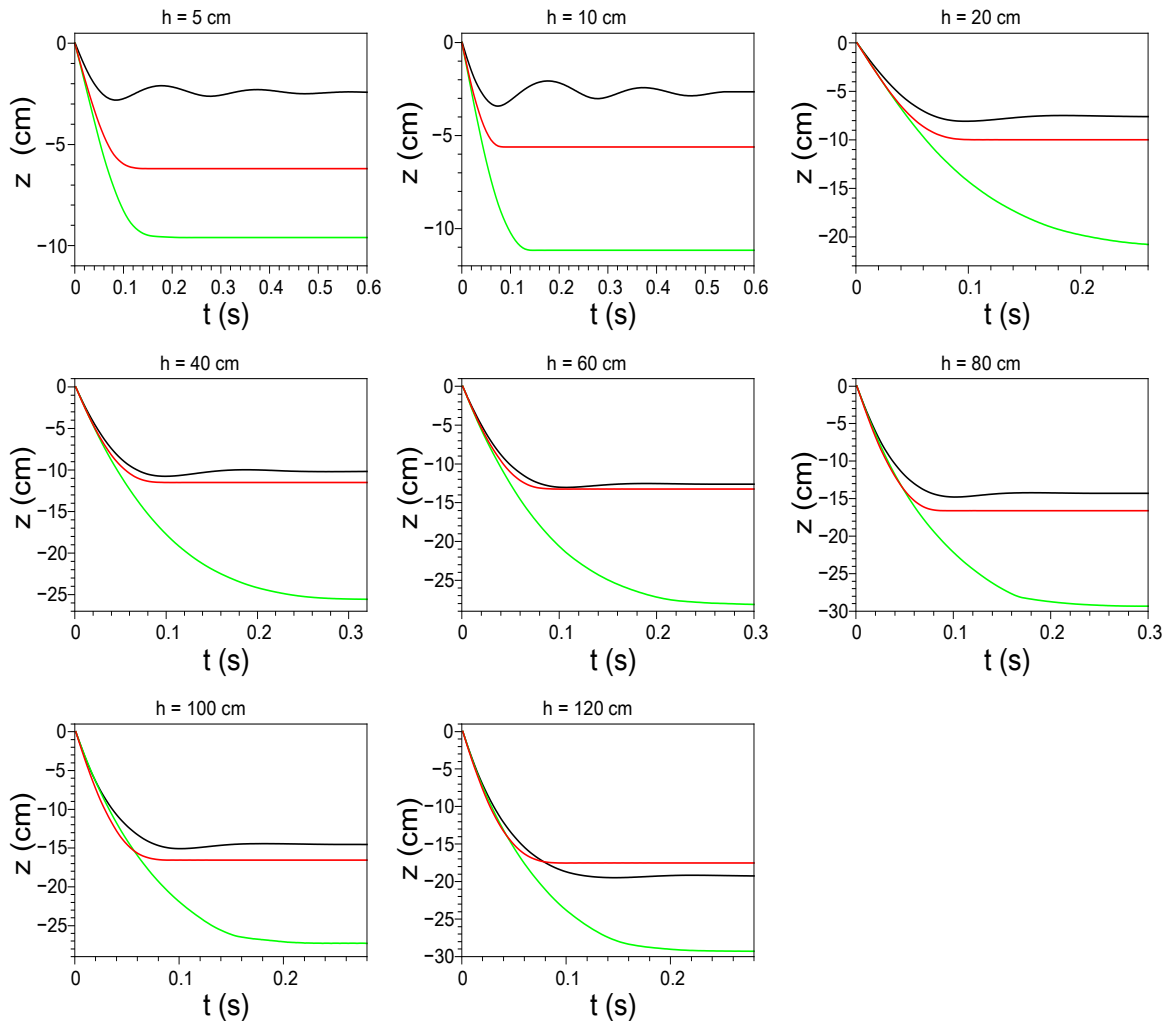
Figura 3.9: Comparación de z vs t de los tres tipos de proyectil impactando desde distintas alturas, el color de la curva representa el tipo de proyectil, la densidad de los proyectiles es \rho_2 = 5.2 \text{ g/cm}^3 . La convención de colores es: negro-repulsivo, verde-neutro y rojo-atractivo.
