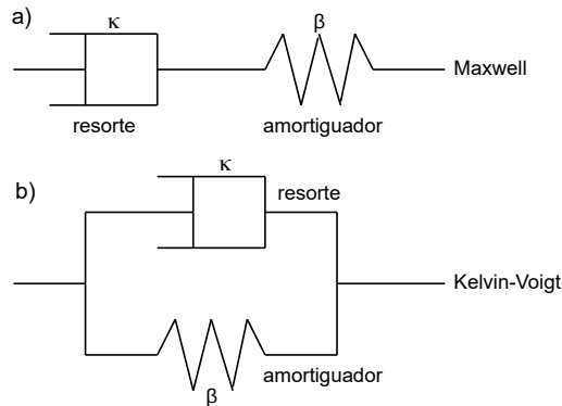
Figura 3.1: Ilustración esquemática de los modelos viscoelásticos clásicos. (a) El modelo de Maxwell consiste en una conexión en serie de un amortiguador y un resorte. (b) El modelo de Kelvin-Voigt consiste en una conexión en paralelo de estos elementos.
