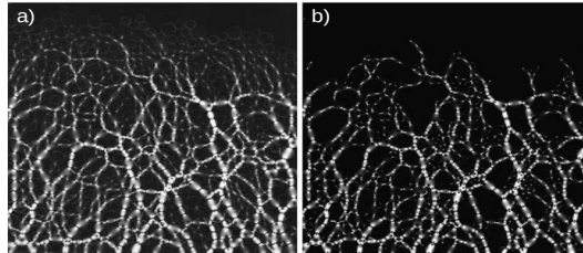
Figura 1.1: Caracterización con discos fotoelásticos de las fuerzas de contacto entre granos. a) Se muestra el resultado experimental y b) las simulaciones correspondientes. Figura tomada de [15].
