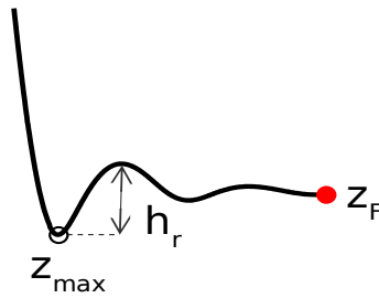
Figura 3.13: Curva representativa z vs t de un proyectil repulsivo. Se muestran los parámetros de medición z_F (profundidad final de penetración), z_{max} (máxima profundidad de penetración) y h_r (altura de rebote).
