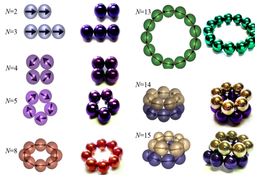
Figura 2.4: Configuraciones de mínima energía en cadenas magnéticas para 2 \leq N \leq 15 . Las configuraciones con flechas negras muestran resultados numéricos del cálculo de energía, mientras que su configuración experimental correspondiente se muestra a la derecha, imágenes obtenidas de [21].
