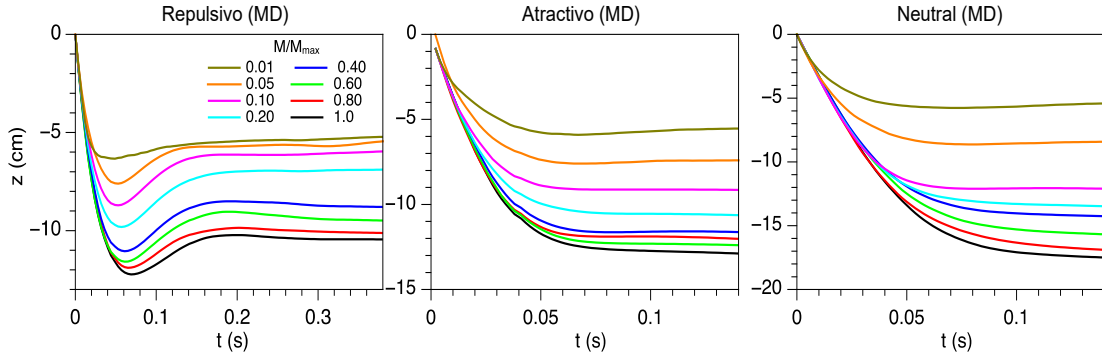
Figura 3.18: Dinámica de penetración obtenida por medio de simulaciones numéricas (MD) para interacciones repulsiva, atractiva y neutra en camas granulares con granos con magnetización M variable.
