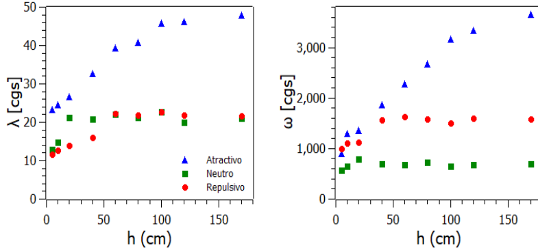
Figura 3.23: Se muestran los parámetros libres \lambda y \omega como función de h para los tres tipos de proyectil. Note que ambos parámetros son considerablemente mayores en el caso del proyectil con interacción atractiva, reflejando que el tamaño efectivo del proyectil aumenta cuando penetra el medio granular.
