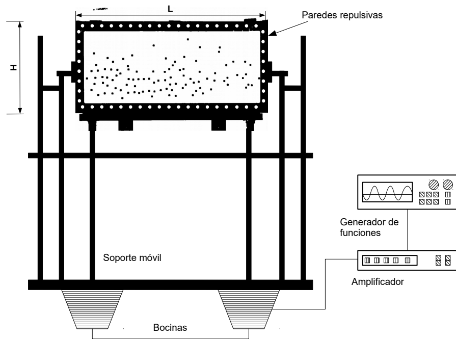
Figura 4.4: Montaje experimental: Sistema granular repulsivo cuasi dos dimensional vibrado verticalmente.
