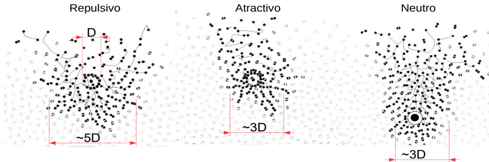
Figura 3.4: Región de perturbación después del impacto de cada proyectil. Se muestran las trayectorias de los granos de la cama granular desplazados debido al impacto.
