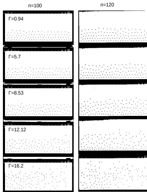
Figura 4.7: Se muestra la dinámica observada experimentalmente con una celda Hele Shaw vibrada verticalmente con granos magnéticos repulsivos en su interior, n representa el número de granos y \Gamma el parámetro de aceleración adimensional.
