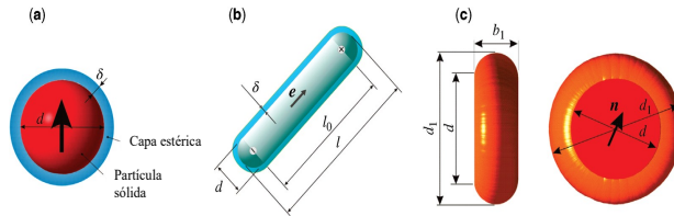
Figura 2.3: Modelación de partículas magnéticas: (a) partícula esférica con un momento dipolar magnético en el centro de la partícula, (b) partícula esfero-cilíndrica con cargas magnéticas norte y sur en ambas hemisferas y (c) partícula tipo disco con momento dipolar magnético en el centro. Imágenes obtenidas de [3].
