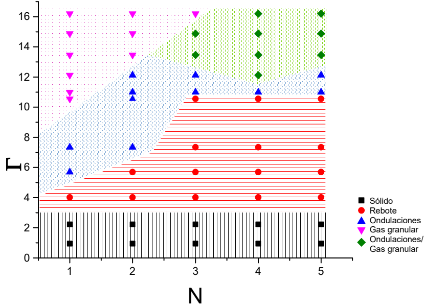
Figura 4.8: Diagrama de fases representativo de un sistema granular bidimensional con interacciones repulsivas vibrado verticalmente. Los cuatro fenómenos explorados cualitativamente en este sistema se indican con diferentes colores. Los valores para hallar la dinámica de sólido, rebote, ondulaciones y gas granular son gobernados por los parámetros \Gamma y N .
