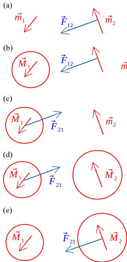
Figura 1.5: Diagrama ilustrando los cinco pasos del argumento con tercera ley de Newton para mostrar que la fuerza entre dos esferas uniformemente magnetizadas es idéntica a la fuerza entre dos dipolos puntuales.
