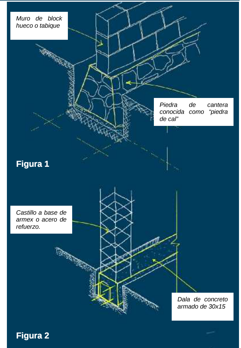
Cimentaciones de la vivienda tradicional en Playa Vicente Ver. Boceto realizado por el autor
