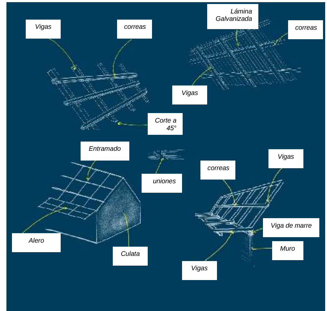
Composición de la cubierta de la vivienda tradicional en Playa Vicente Ver. Boceto realizado por el autor
