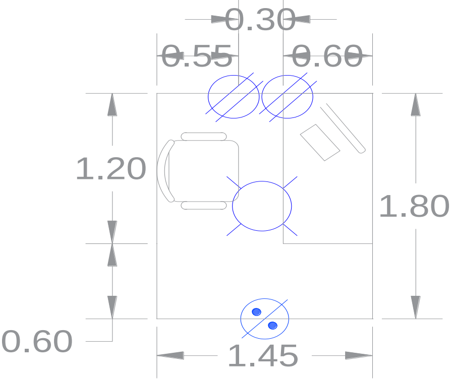
Módulo de cubículos con instalación eléctrica propuesta en planta.
