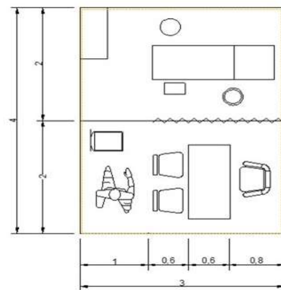
Módulo del consultorio médico en planta.
