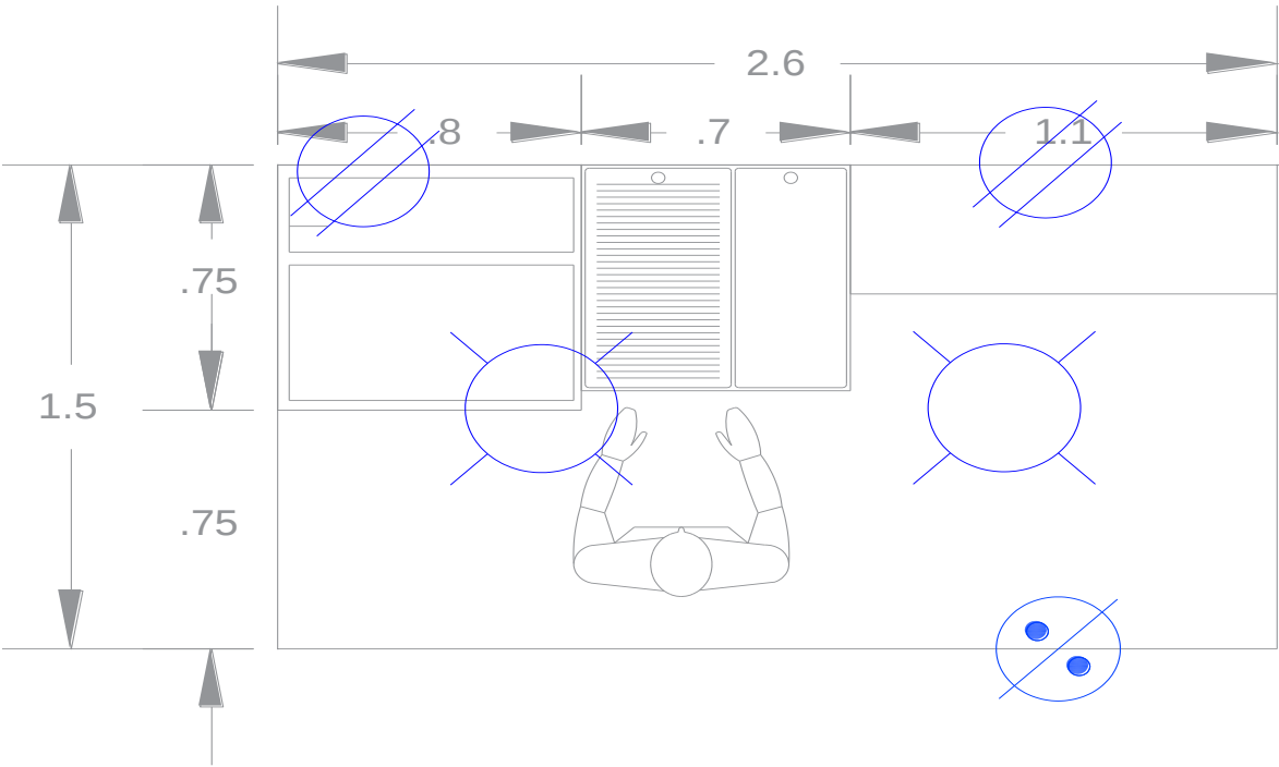
Módulo de lavandería con instalación eléctrica propuesta en planta.
