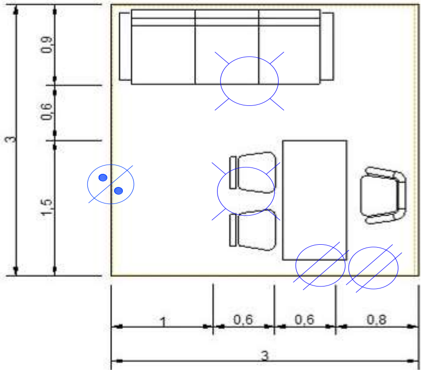
Módulo de consultorio psicológico con instalación eléctrica propuesta en planta.
