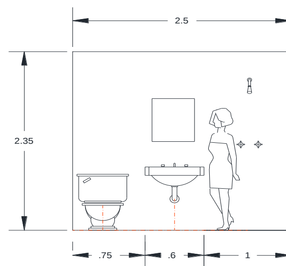
Módulo baño en alzado.
