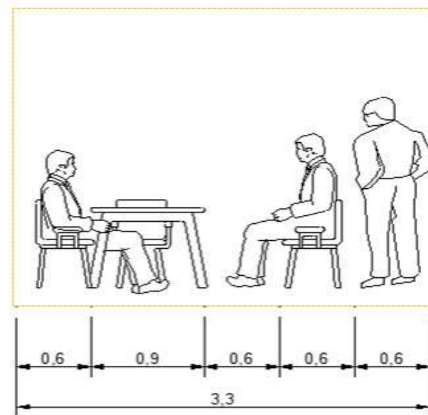
Módulo de una mesa del comedor en alzado.
