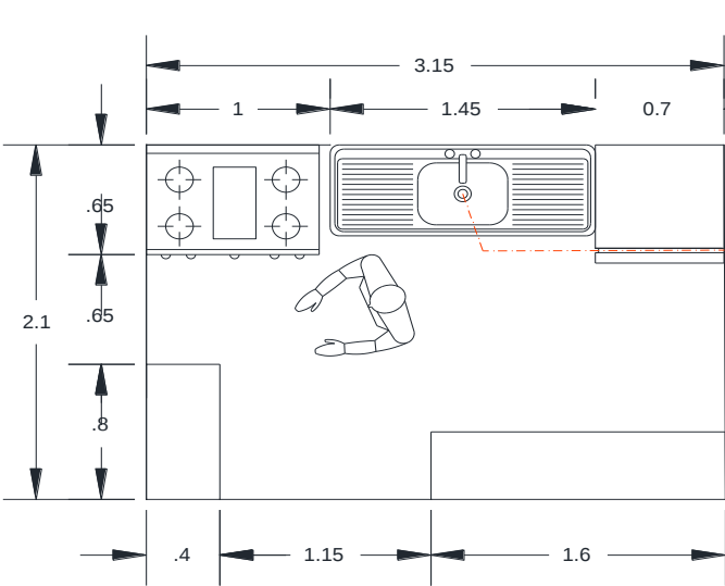
Módulo de cocina en planta.
