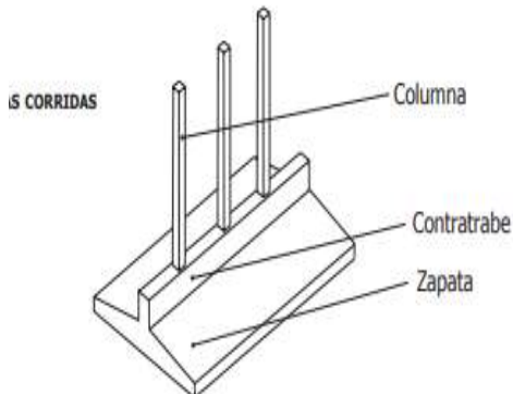
Tipos de cimentación recomendadas
