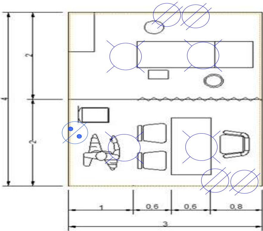
Módulo de consultorio médico con instalación eléctrica propuesta en planta.
