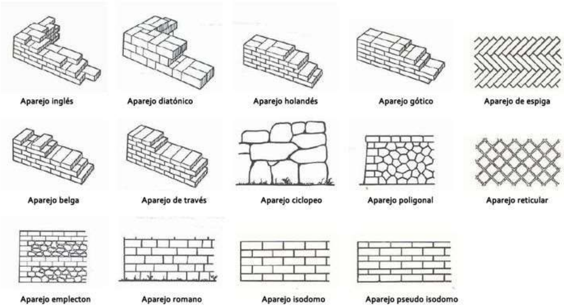
Tipos de muros
