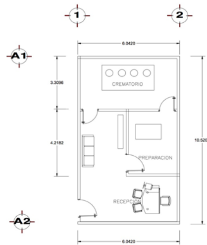
PLANTA CREMACIÓN
