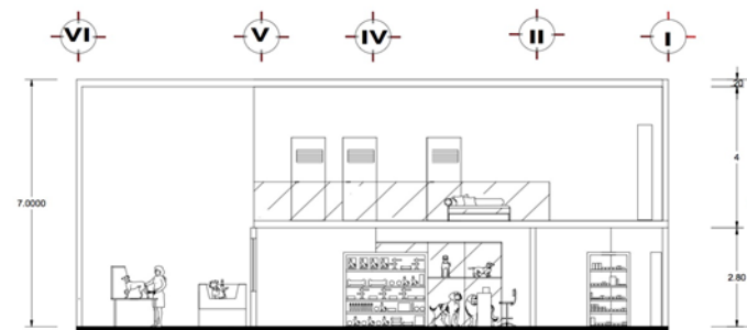
CORTE A-A
