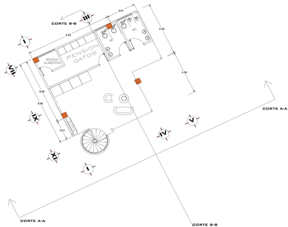
PLANTA ALTA PENSION
