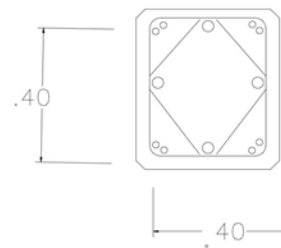
COLUMNA 2
