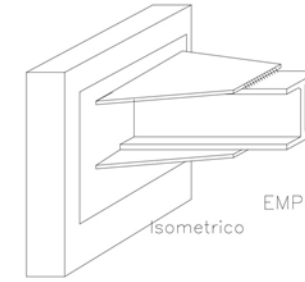
EMPOTRAMIENTO EN COLUMNA DE ACERO
