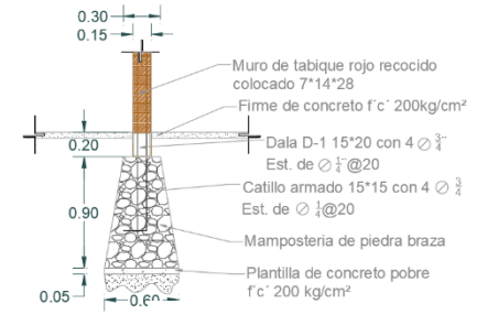
Cimentación central zapata corrida de mamposteria
