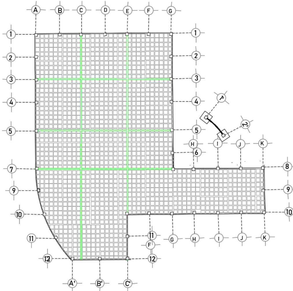
Cimbra de Columnas y vista de de armado de losa.
