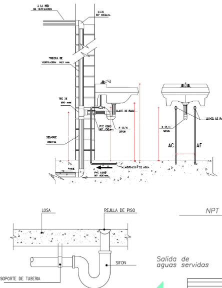
CORTE
