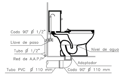
CORTE
