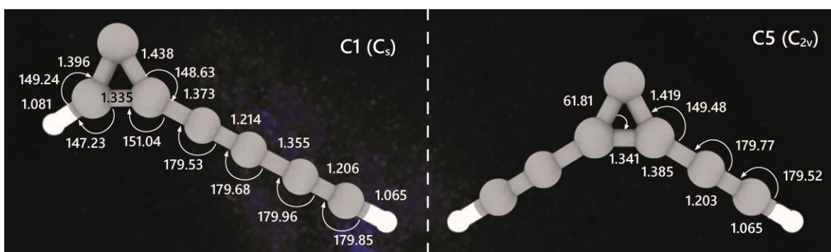
5.1.2. Geometrías optimizadas de los complejos de colisión C1 y C5. Los complejos de colisión optimizados a nivel de teoría APFD/6-311+G(2d,p). Los grupos puntuales se muestran entre paréntesis, las distancias de enlace están en Å y los ángulos de valencia en grados.
