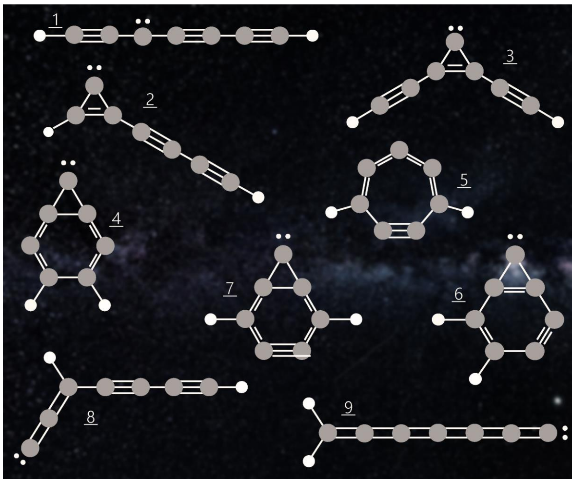
Figura 1.4.2. Estructuras calculadas por Thimmakondy y Karton (2017). [146] Se muestran los 9 isómeros empleados en su estudio.
