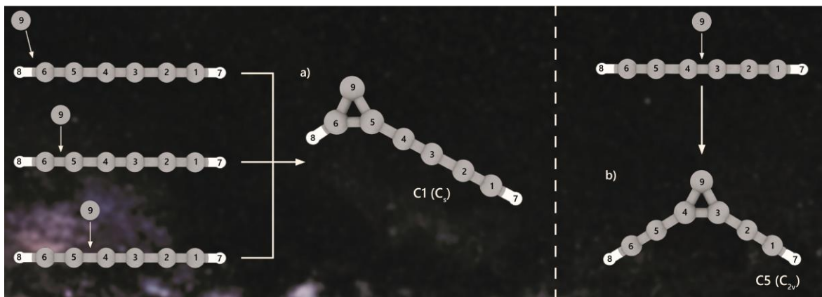
Figura 5.1.1. Simulación de la reacción entre la molécula lineal \text{HC}_6\text{H} y el átomo de C. Complejos de colisión denominados a) C1 y b) C5. El grupo puntual correspondiente se indica entre paréntesis.
