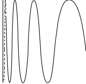
Figura 1.1: El continuo seno (1/x)
