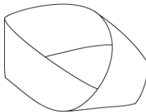
Figura 1.5: Banda de Moebius
