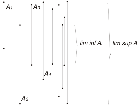
Figura 1.6: Límite superior y límite inferior de una sucesión
