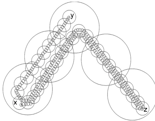
Figura 1.4: X = \bigcap_{n=1}^{\infty} (\bigcup \mathcal{C}_n) es un continuo
