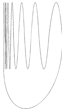
Figura 1.3: Circunferencia de Varsovia
